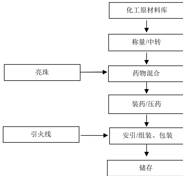
图 2-1：喷花类（花筒/组合型喷花）产品生产工艺流程图
