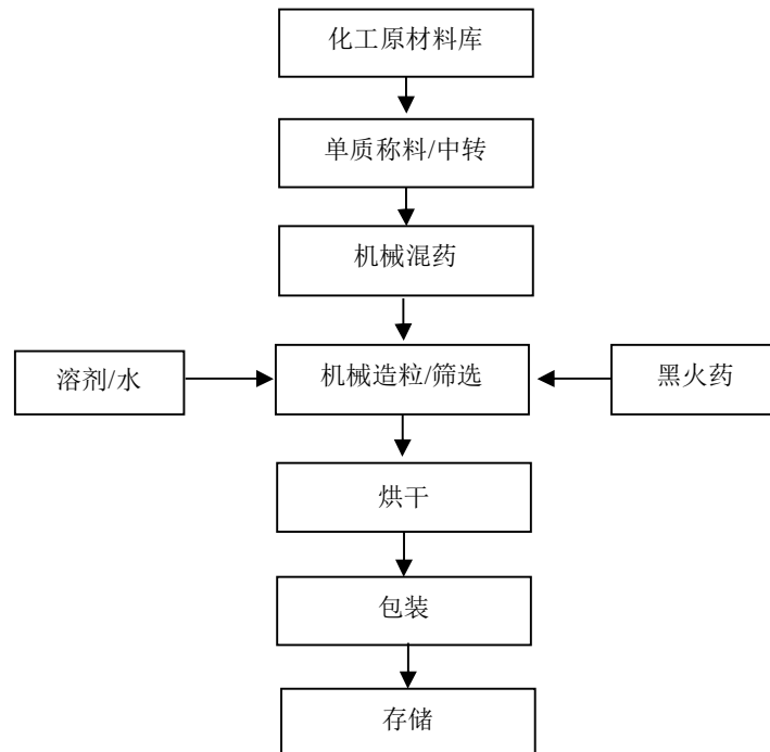
图 2-9：亮珠生产工艺流程图
