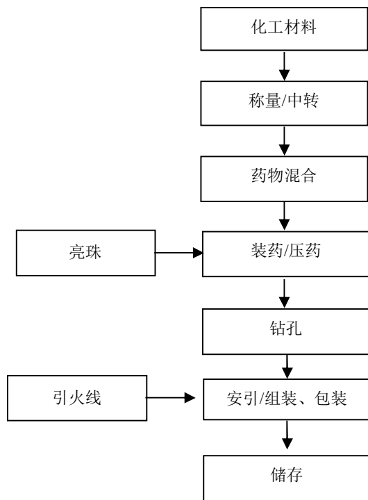
图 2-4：旋转类生产工艺流程图
