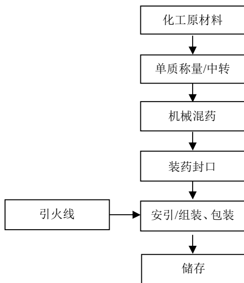
图 2-5：玩具类（线香型-晨光花）生产工艺流程图
