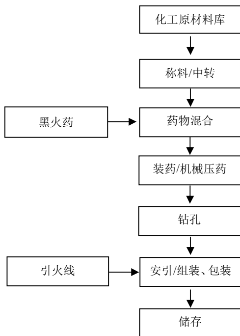
图 2-7：升空类（旋转升空烟花）生产工艺流程图
