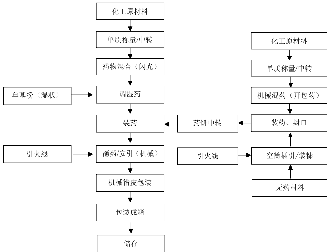
图 2-3：喷花类（闪光炮）生产工艺流程图
