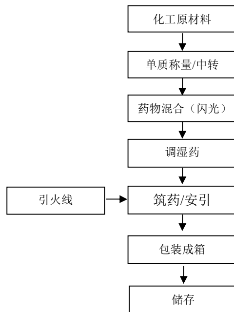
图 2-2：喷花类（闪光）生产工艺流程图
