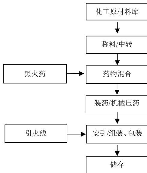
图 2-8：升空类（火箭）生产工艺流程图
