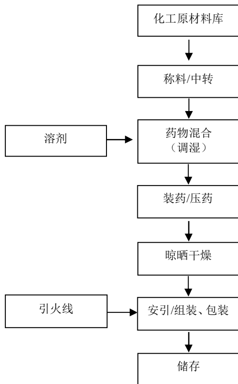
图 2-6：玩具类（玩具造型）生产工艺流程图
