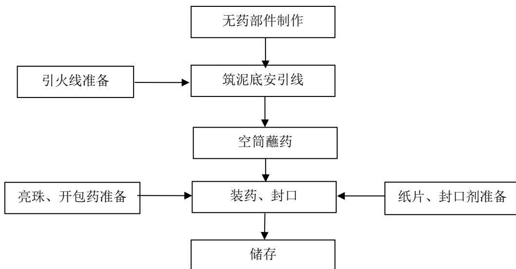
图 2.4-2 内筒效果生产工艺流程图
