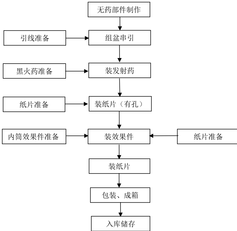
图 2.4-3 组合烟花类产品生产工艺流程图
