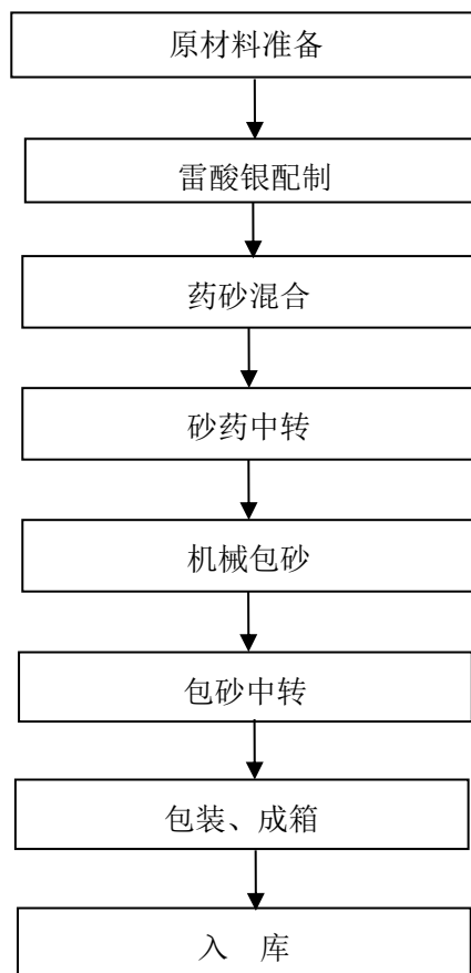
图 2.4-6 玩具类（摩擦型/砂炮）产品生产工艺流程图
