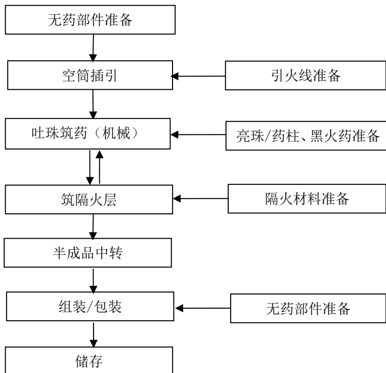
图 2.4-4 吐珠类（药粒/柱型）产品生产工艺流程图
