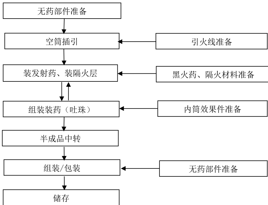
图 2.4-5 吐珠类（内筒型）产品生产工艺流程图
