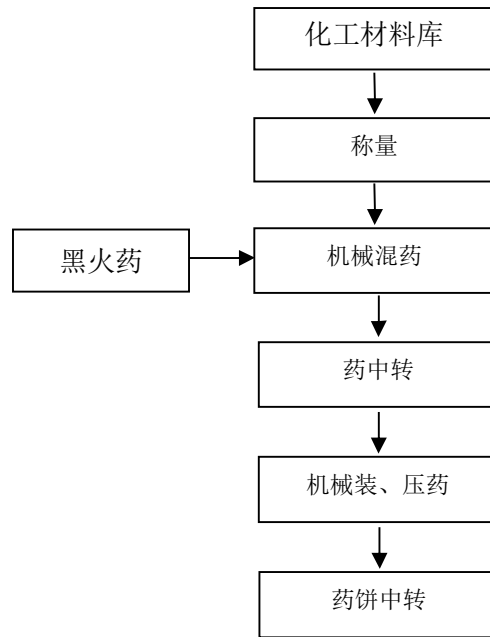
图 2-2：笛音效果件生产工艺流程图
