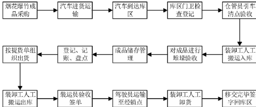
图 2.8 烟花爆竹产品经营工艺流程图
