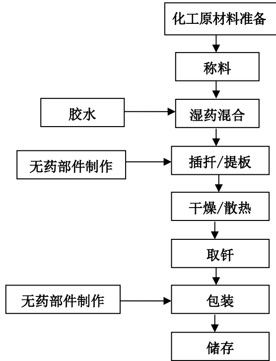
图 2.4-4 玩具类（线香型/电光型）生产工艺流程图
