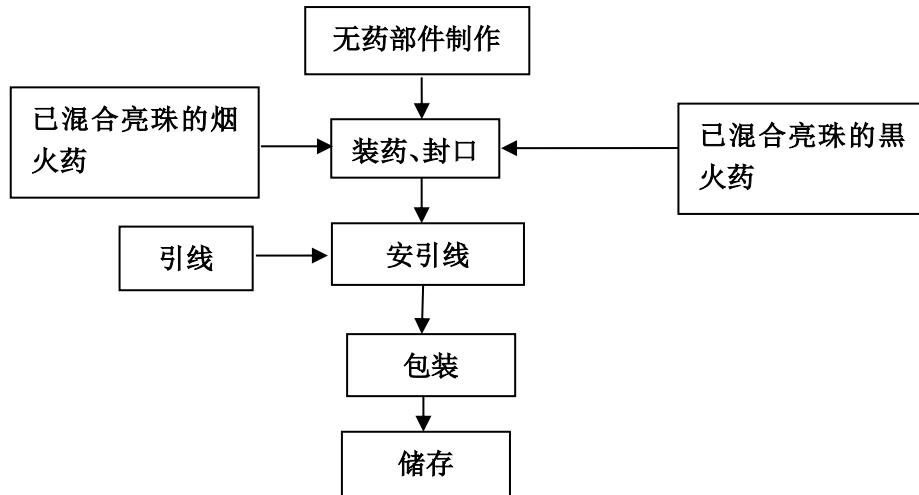
图 2.4-5 喷花类生产工艺流程图
