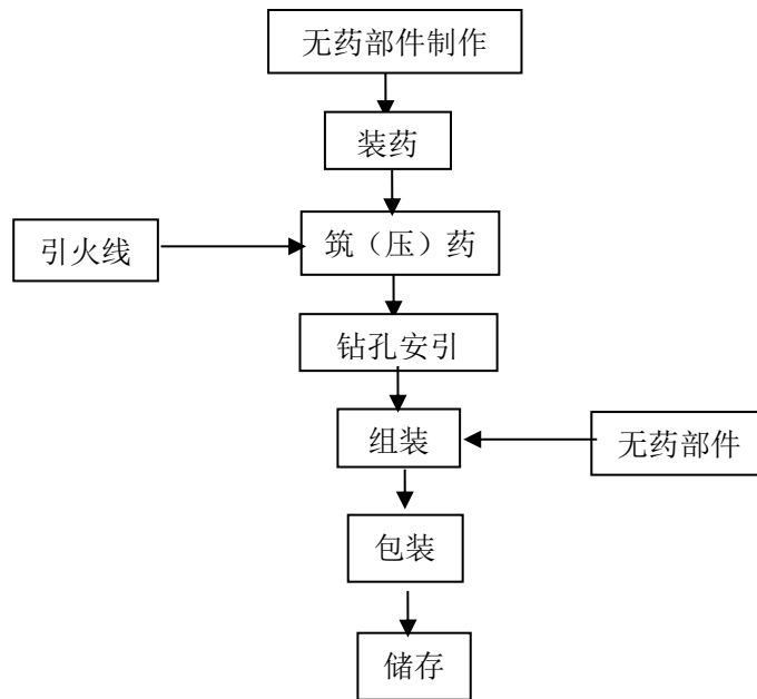
图 2.4-2 旋转类（无轴、有轴）生产工艺流程图
