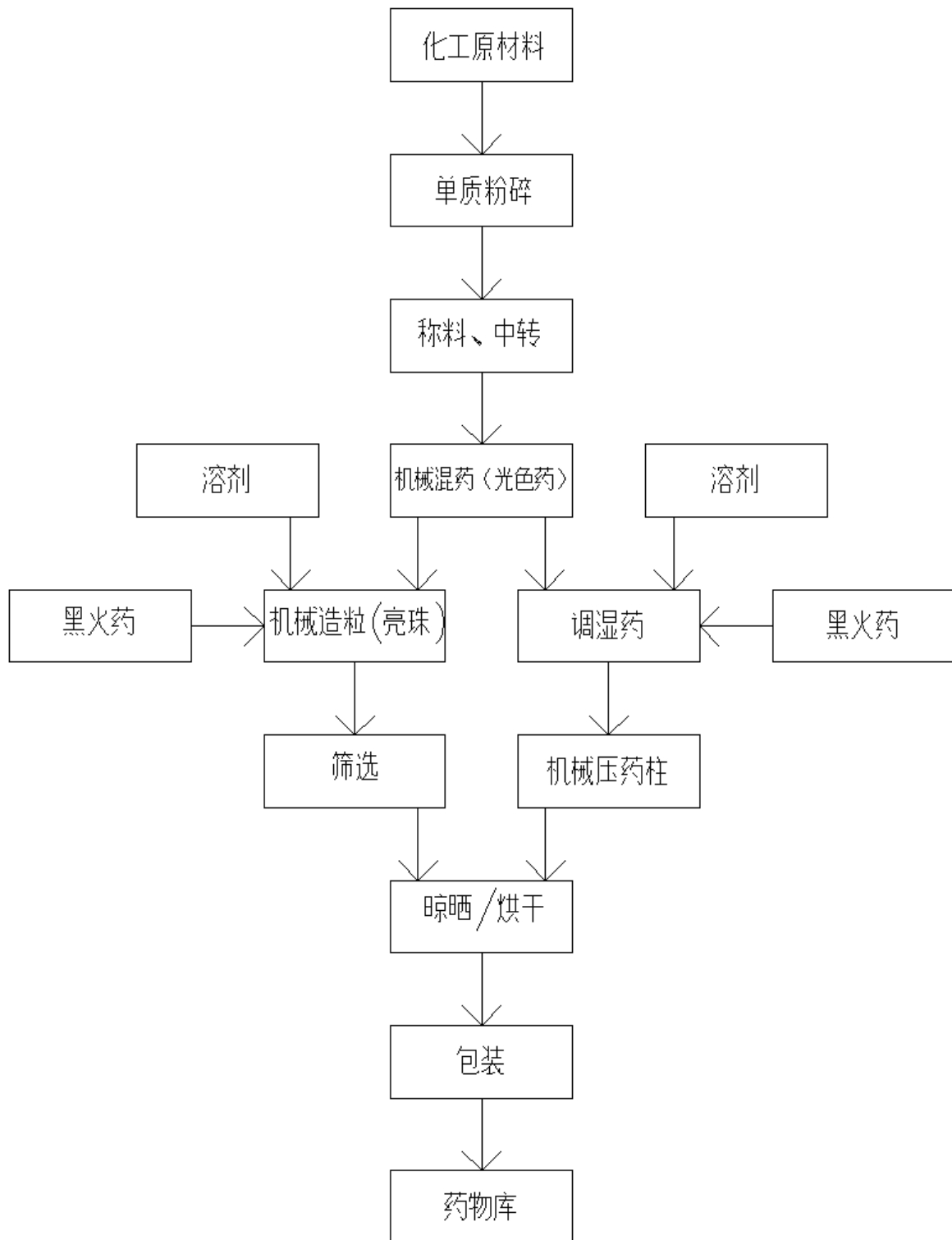
图 2-3 烟火药（亮珠/药柱）生产工艺流程图
