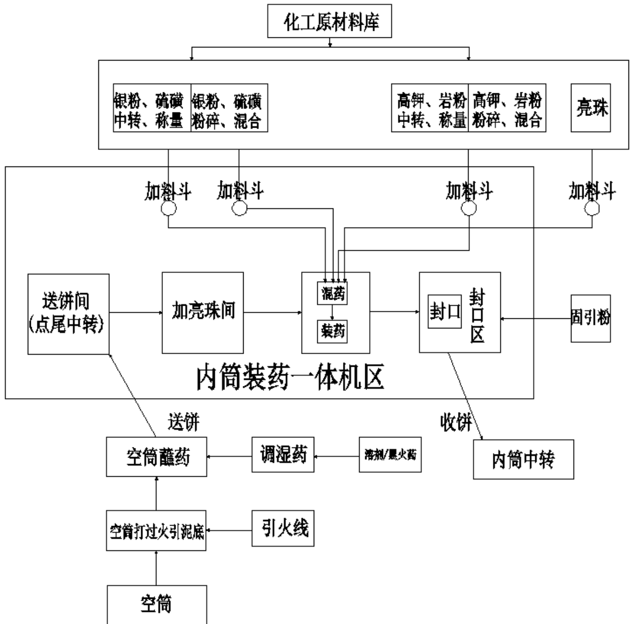
图 2-2 内筒机械装药一体机生产工艺流程图
