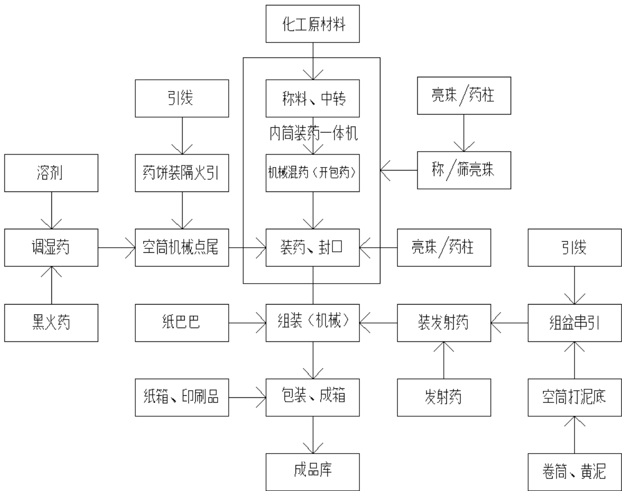
图 2-1 组合烟花类生产工艺流程图
