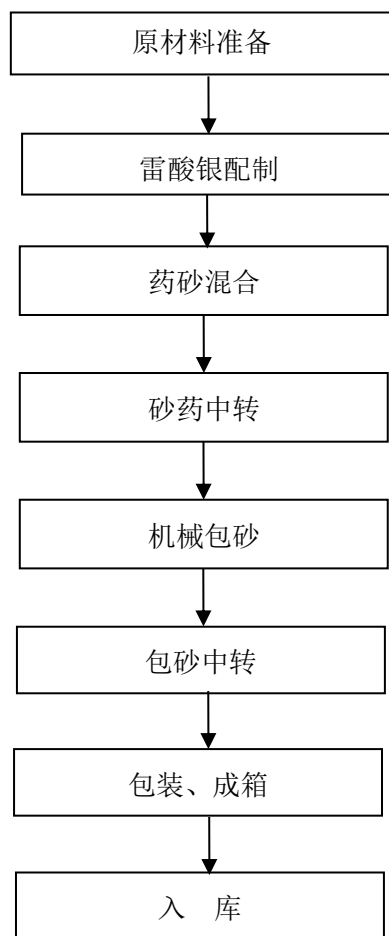
图 2.6-2 玩具类（摩擦型/砂炮）产品生产工艺流程图
