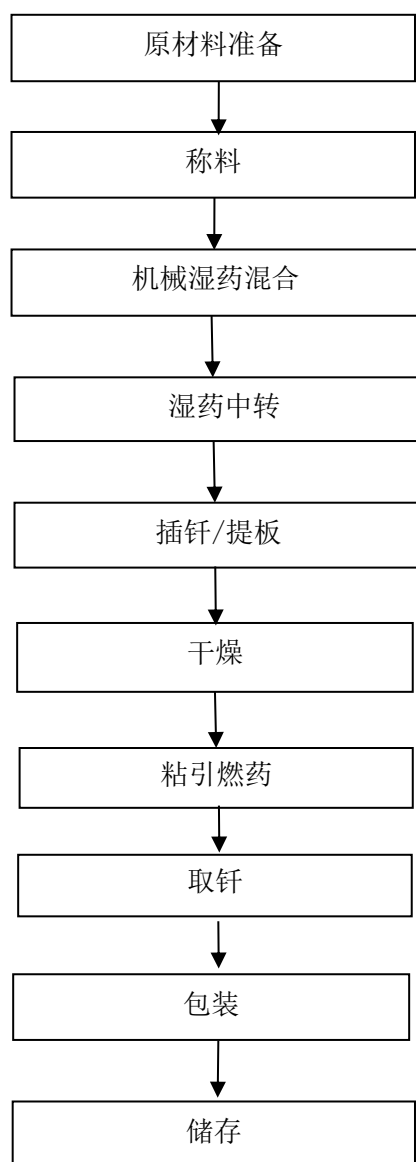
图 2.6-1 玩具类（线香型/电光花）产品生产工艺流程图
