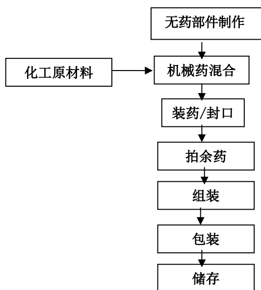
图 2-6-4 玩具类（线香型/晨光花）生产工艺流程图
