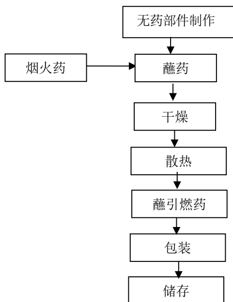
图 2-6-3 玩具类（线香型/涂敷型）生产工艺流程图
