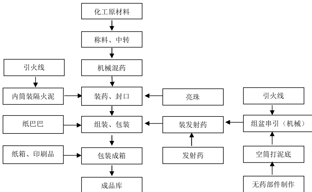
图 2-1：组合烟花类生产工艺流程图
