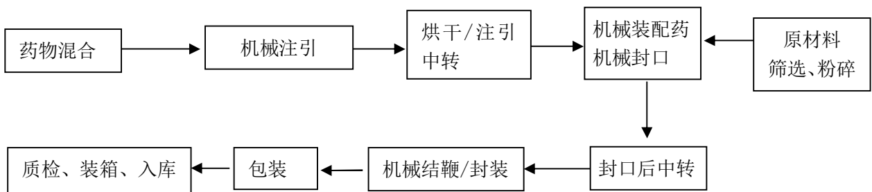
图 2-3：爆竹生产（注引）工艺流程图
