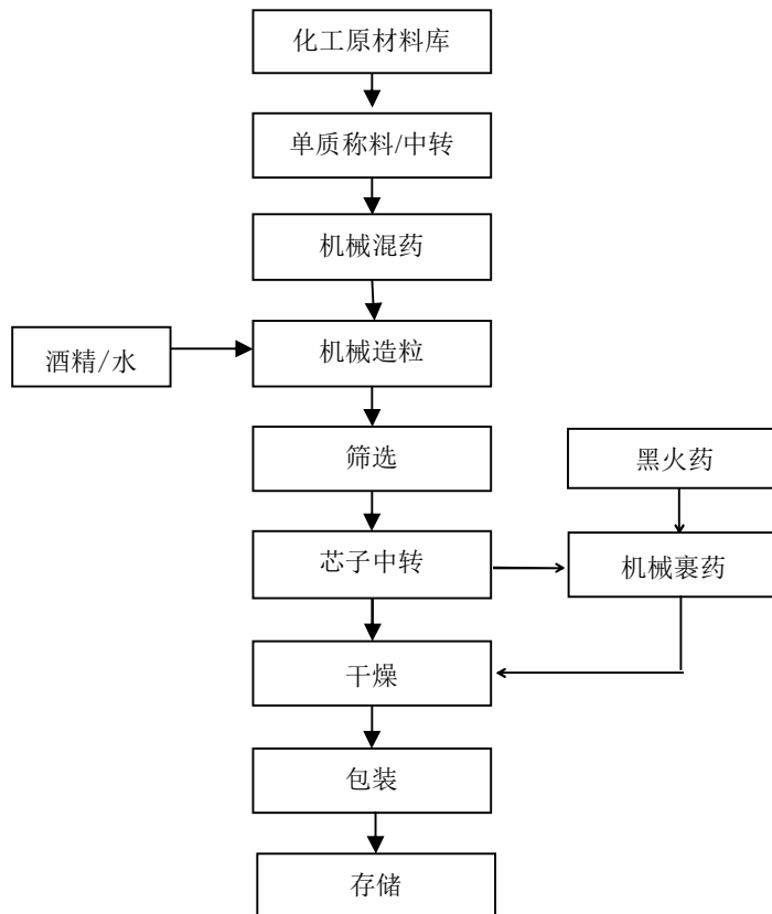
图 2-4：亮珠生产工艺流程图
