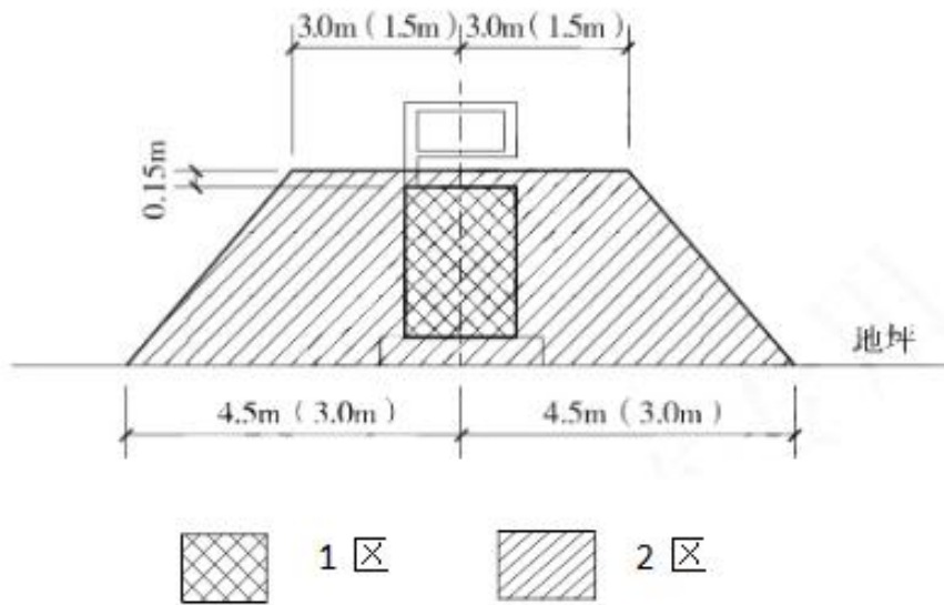
图3.11-2 汽油加油机爆炸危险区域划分
