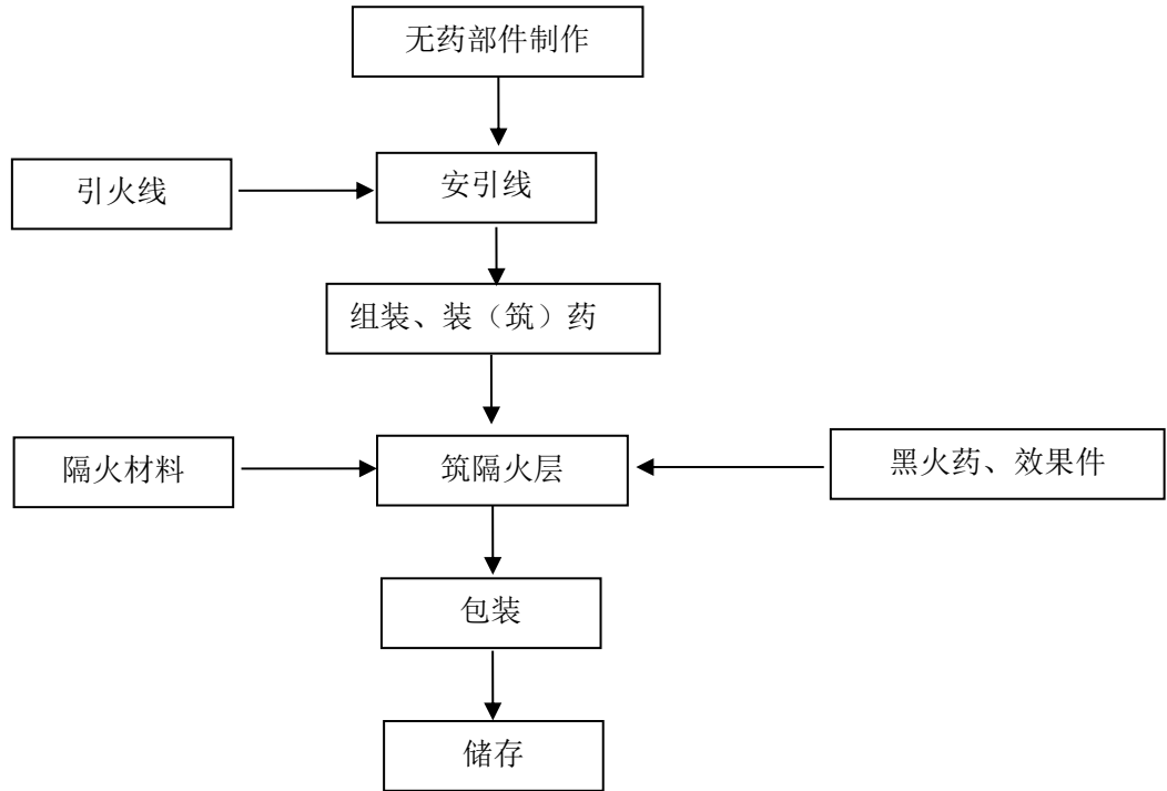
图 2.4-4 吐珠类产品生产工艺流程
