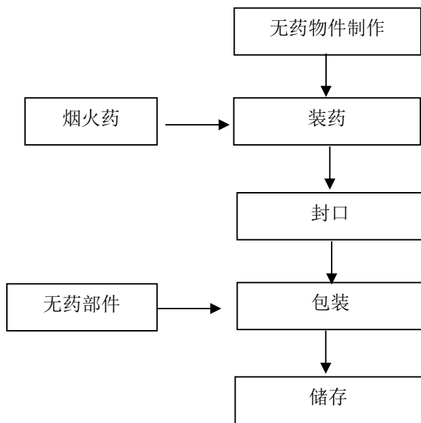
图 2-4-5 玩具类（晨光花）生产工艺流程图
