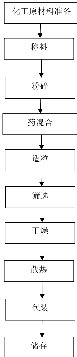
图 2.4-1 亮珠生产工艺流程图
