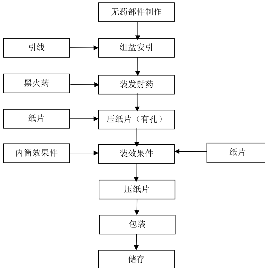
图 2.4-2 效果内筒生产工艺流程图
