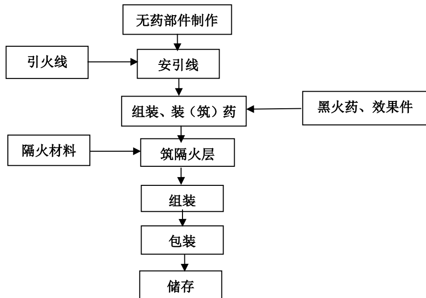
图 2-4-1 吐珠类产品生产流程图
