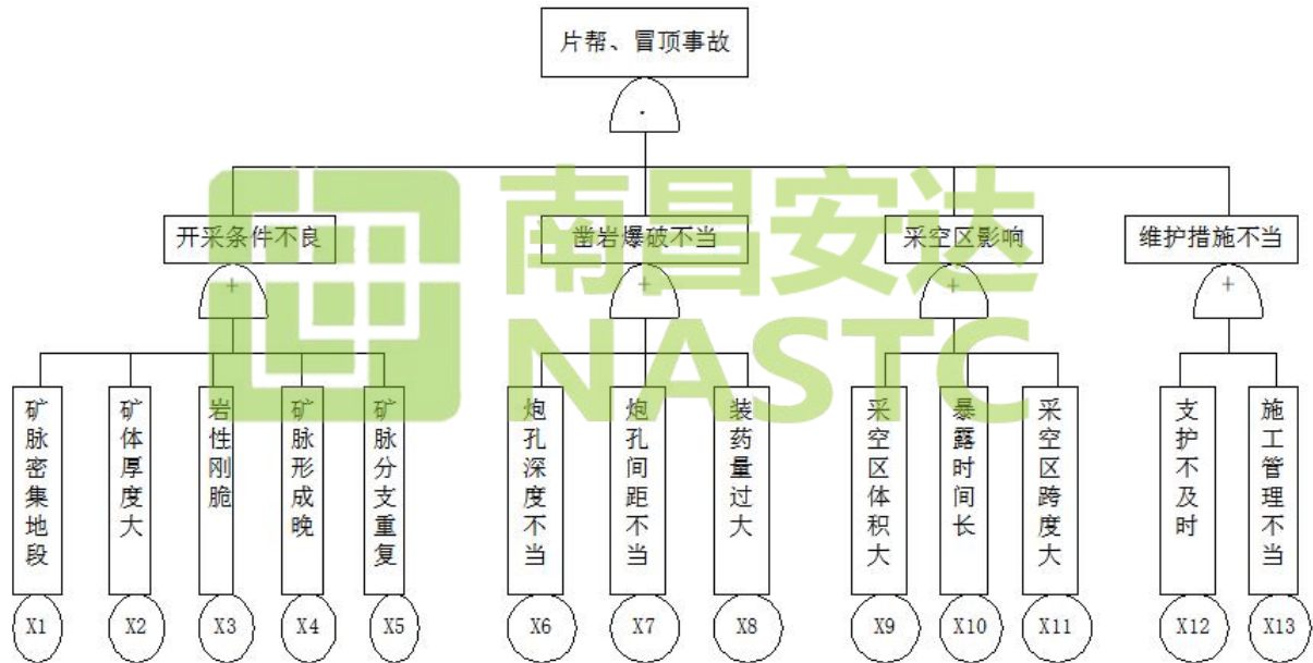
图 5.2-2 采矿过程中片帮、冒顶事故树
