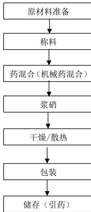
图 2.4-2 引线药生产工艺流程图
