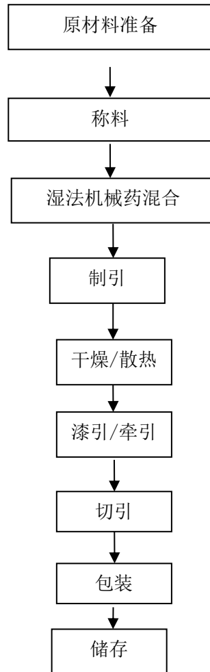
图 2.4-1 湿法制安引产品生产工艺流程图
