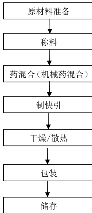
图 2.4-4 快引生产工艺流程图
