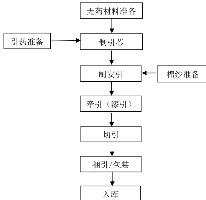
图 2.4-3 引火线（安全引火线）产品生产工艺流程图
