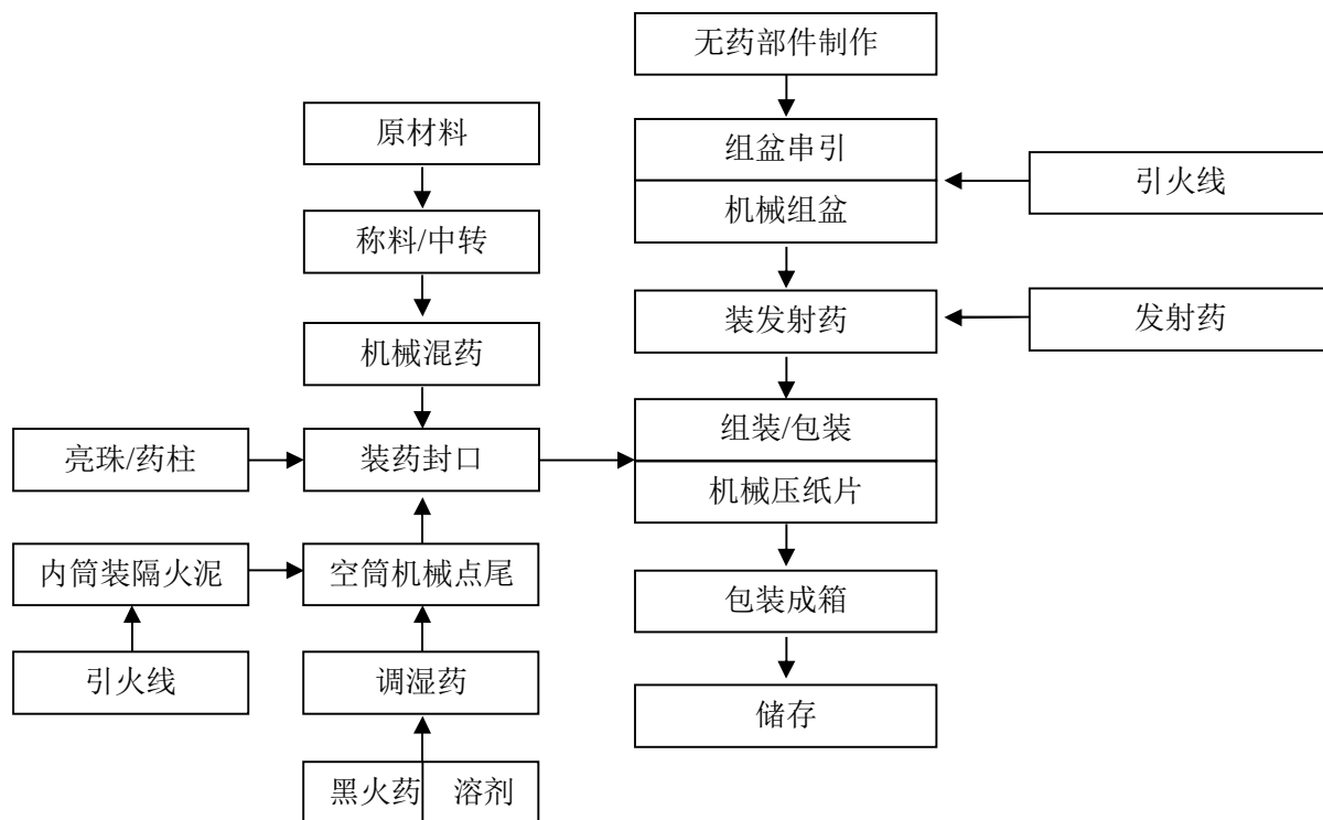
图 2-1：组合烟花类产品生产工艺流程图
