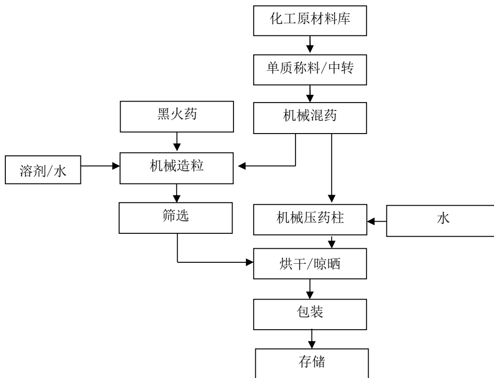
图 2-2：亮珠/药柱生产工艺流程图
