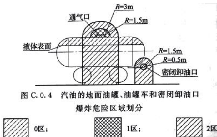
图 3.9-3 油罐车卸汽油爆炸危险区域
