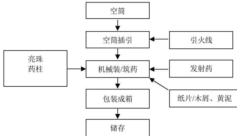
图 2-1：C 级吐珠生产工艺流程图
