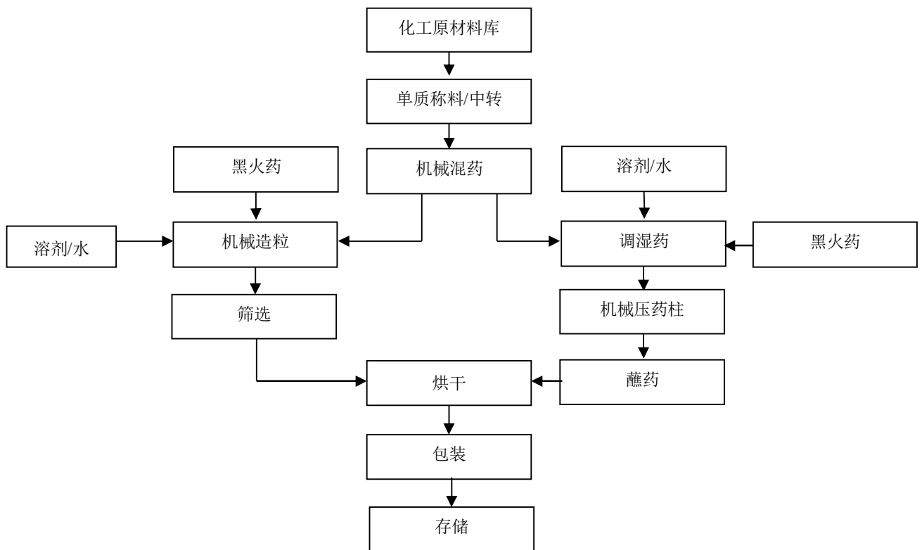
图 2-2：亮珠/药柱生产工艺流程图
