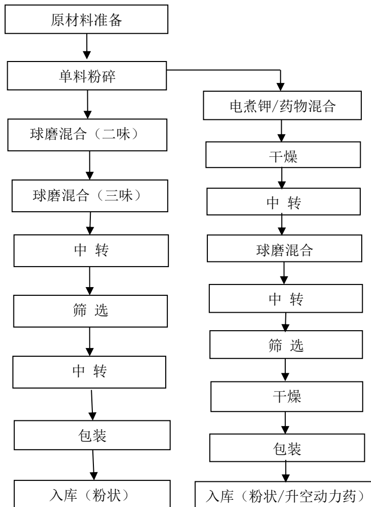
图 2.4-1 黑火药（粉状）产品生产工艺流程图
