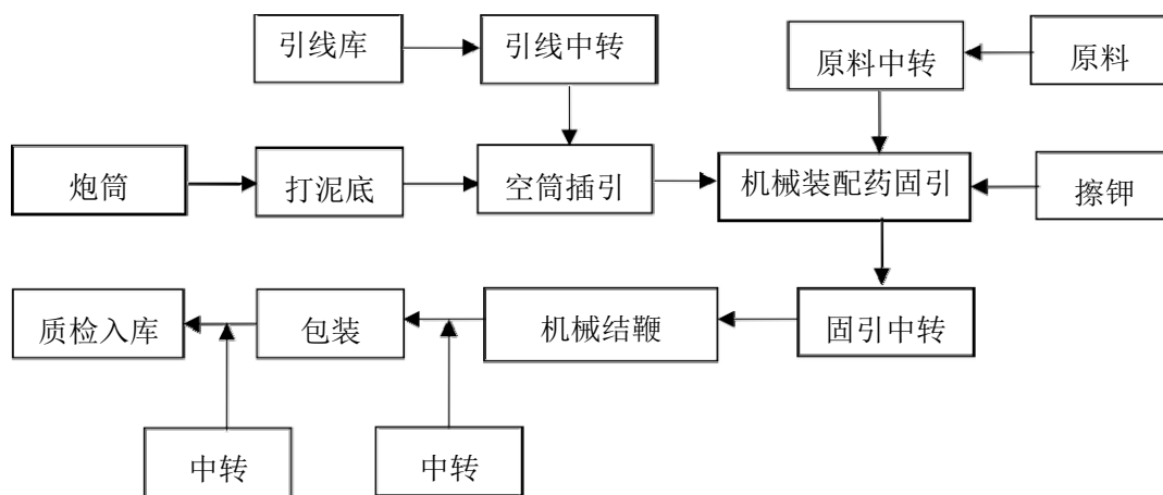
图 2.4-1 爆竹生产工艺流程示意图
