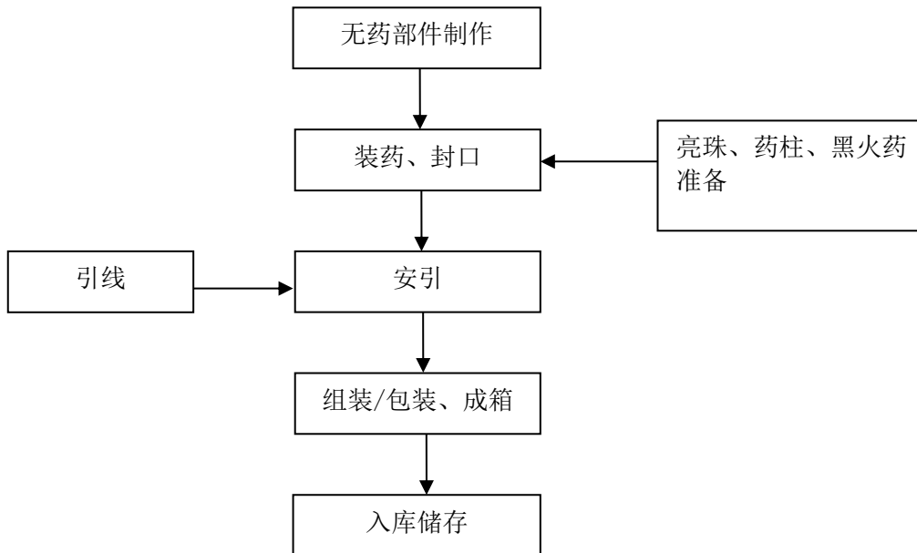
图 2.4-4 喷花类产品生产工艺流程图
