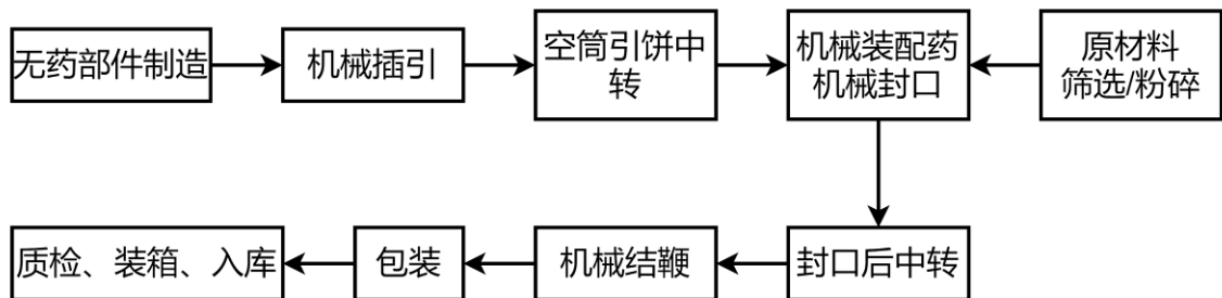
图 2-1: 爆竹生产工艺流程
