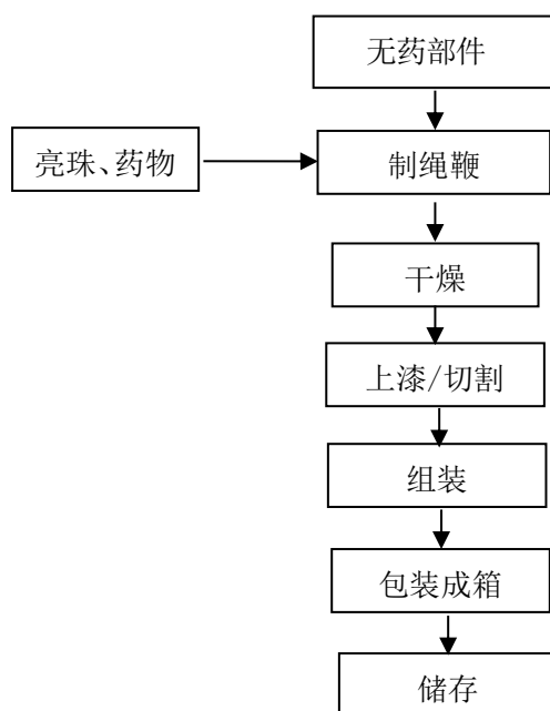
图 2-4-2 玩具类（线香型/绳鞭）生产工艺流程图
