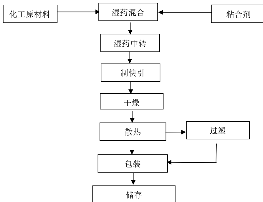
图 2-4-1 线引产品生产工艺流程图
