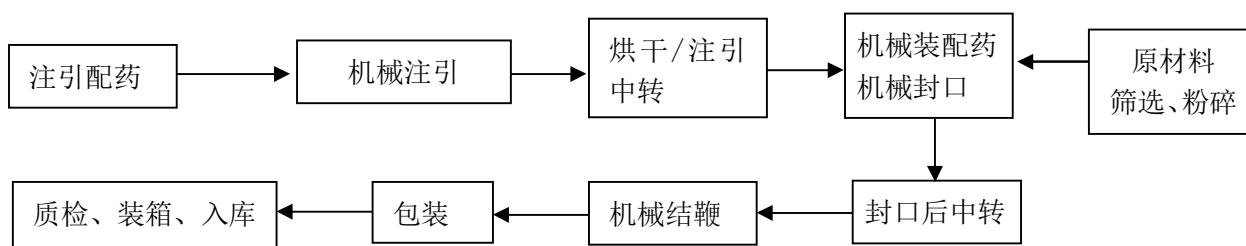
图 2-2：爆竹生产（注引）工艺流程图
