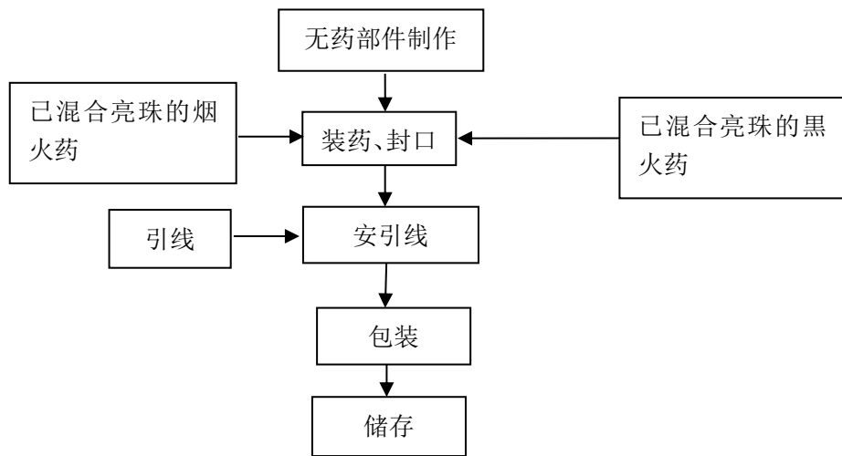
图 2-4-3 组合烟花产品生产工艺流程图
