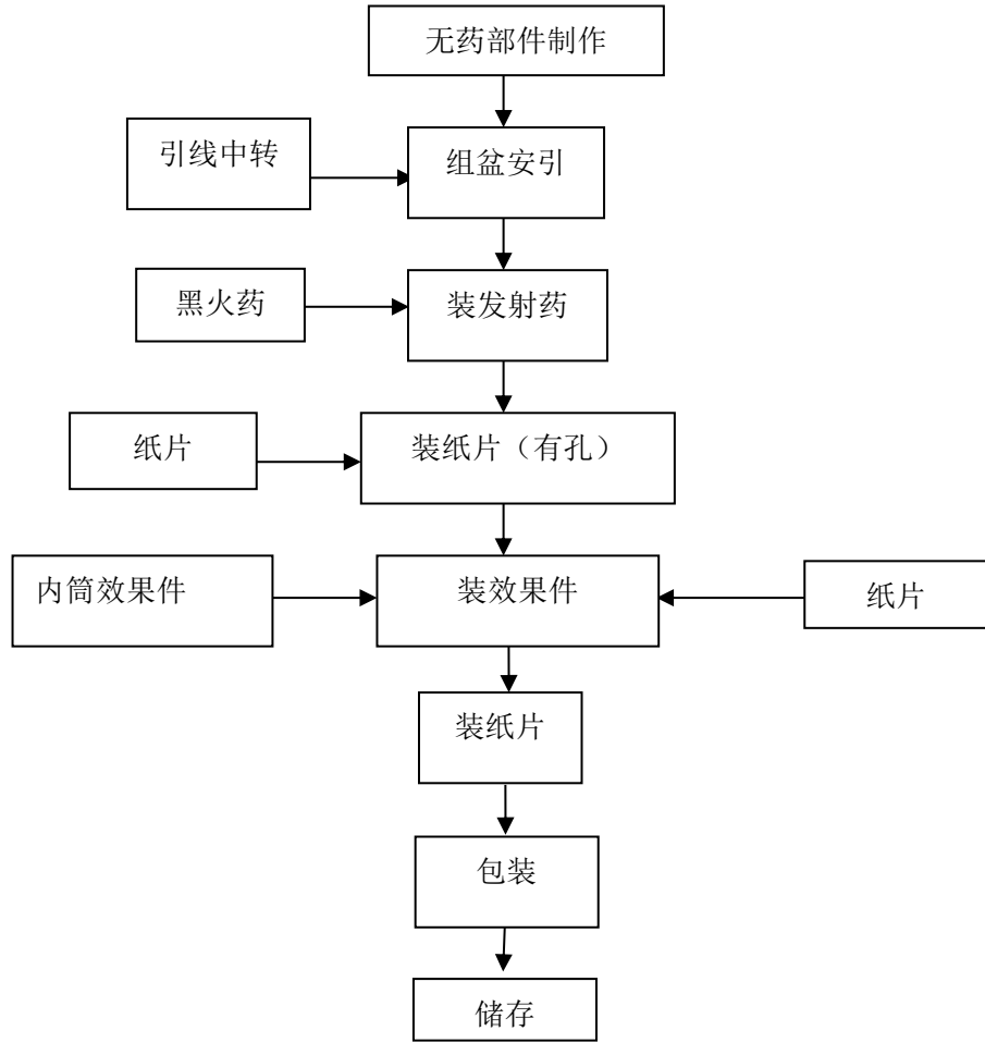
图 2-4-3 组合烟花产品生产工艺流程图
