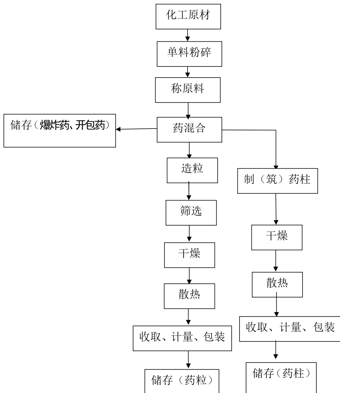
图 2.3-1 药物裸药效果件生产工艺流程图（药粒、药柱）
