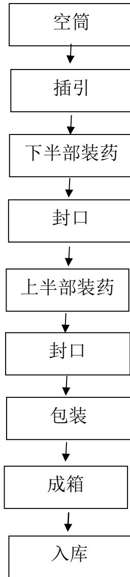
图 2.3-4 升空类（双响）生产工艺流程图
