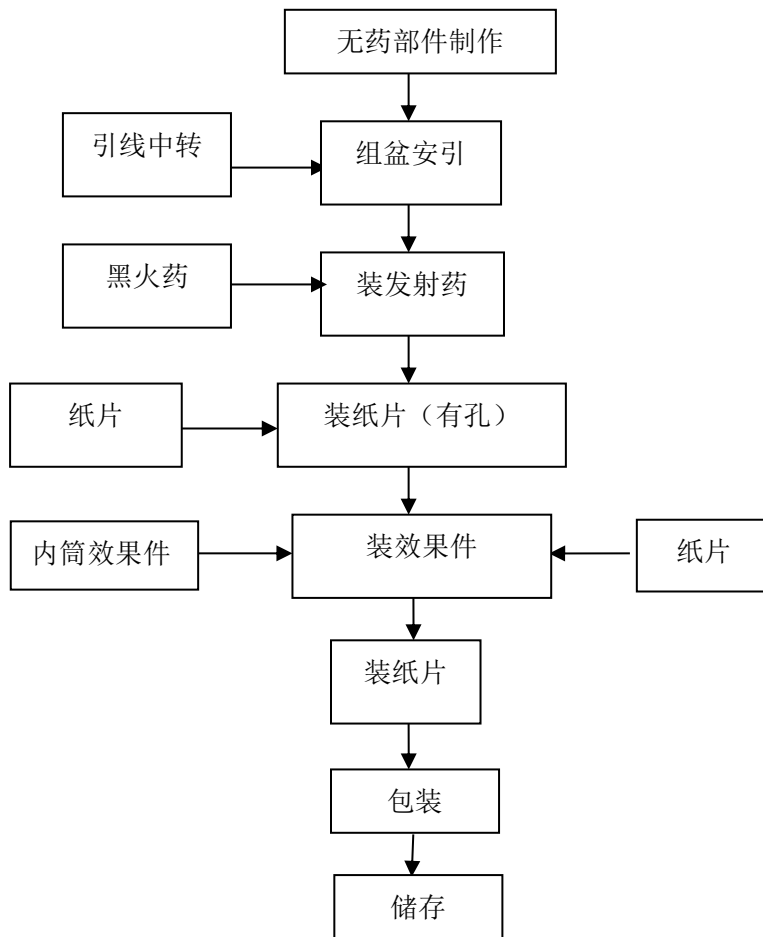
图 2-4-2 效果内筒生产流程图
