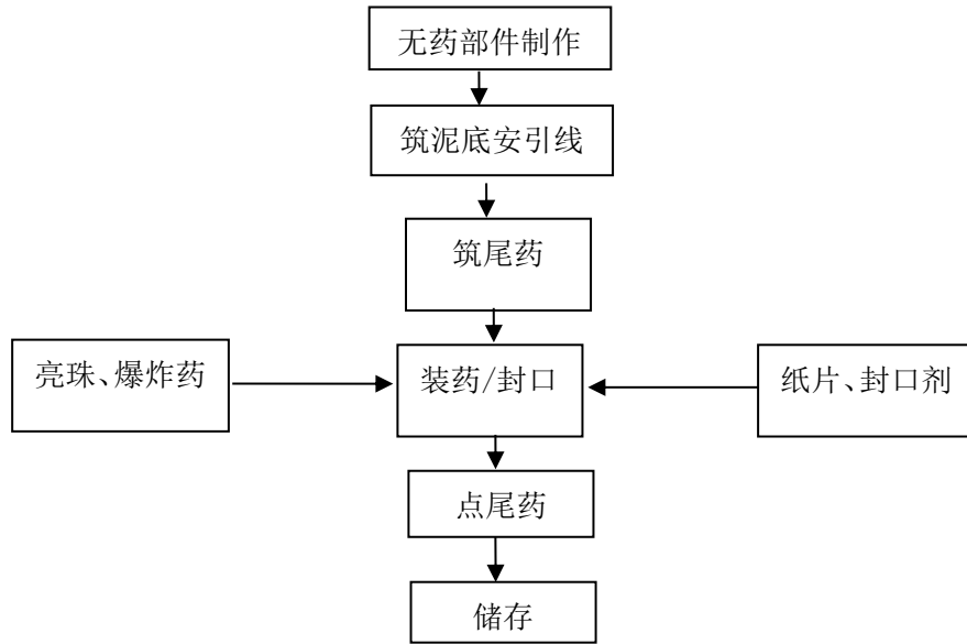
图 2-4-2 效果内筒生产流程图
