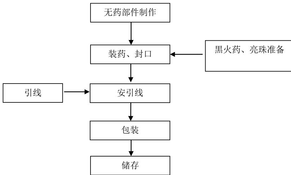
图 2.4-4 喷花类产品生产流程图
