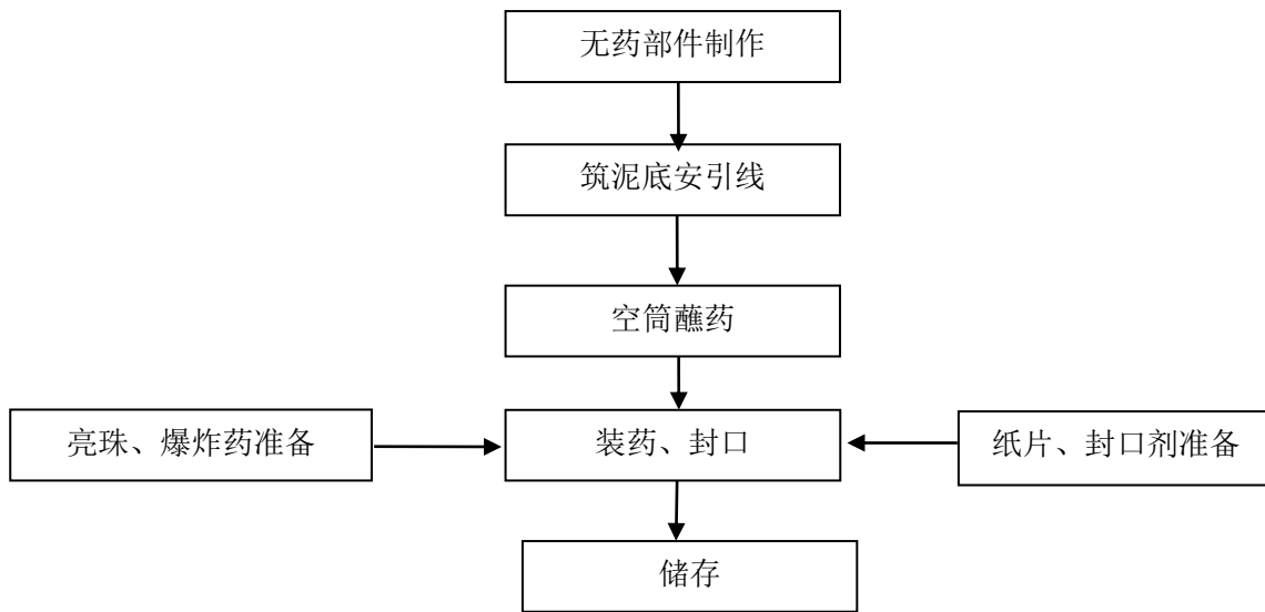
图 2.4-2 效果内筒生产工艺流程图
