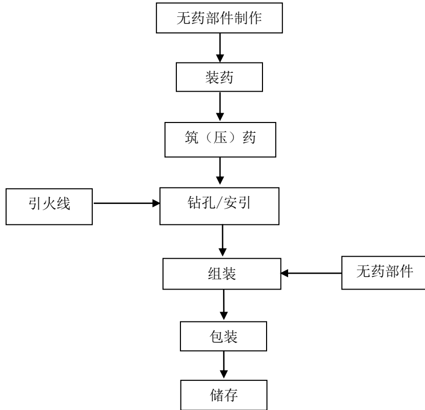
图 2.4-6 升空类（旋转升空）生产工艺流程图
