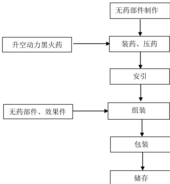
图 2.4-7 升空类（火箭）产品生产流程图
