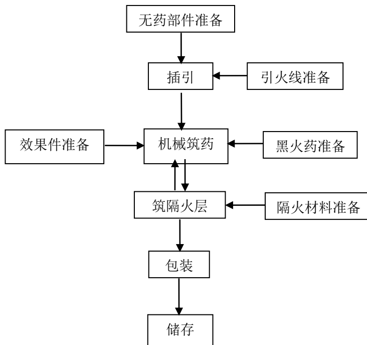
图 2.4-5 吐珠类产品生产工艺流程图
