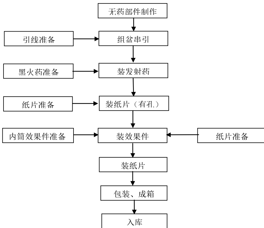
图 2.6-3 组合烟花类产品生产工艺流程图
