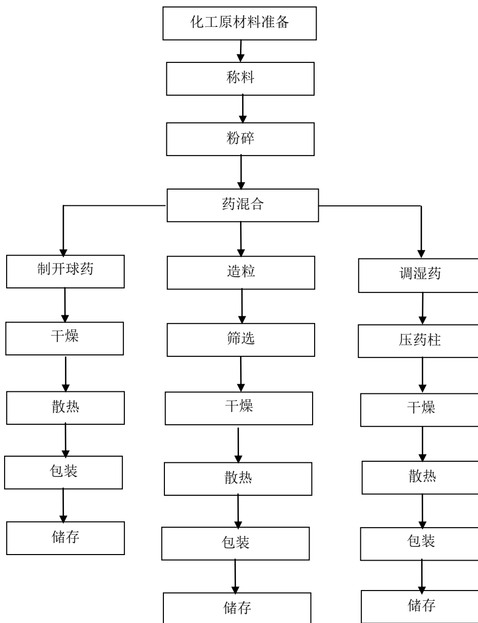
2.6-2 亮珠、开球药、药柱生产工艺流程图
