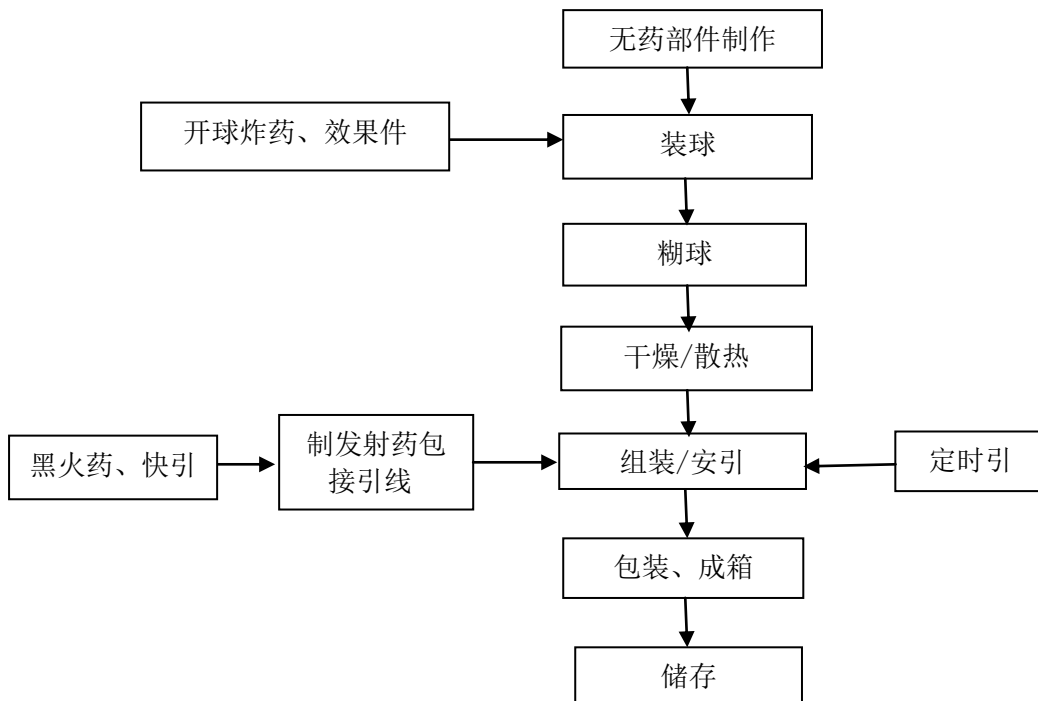
图 2.6-4 礼花类（小礼花）产品生产工艺流程图
