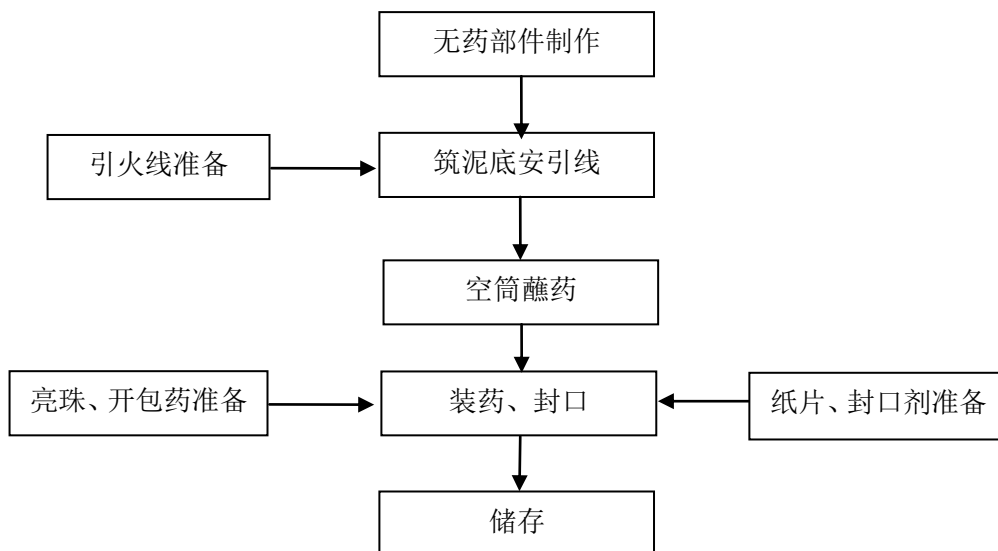
图 2.6-1 效果内筒生产工艺流程图
