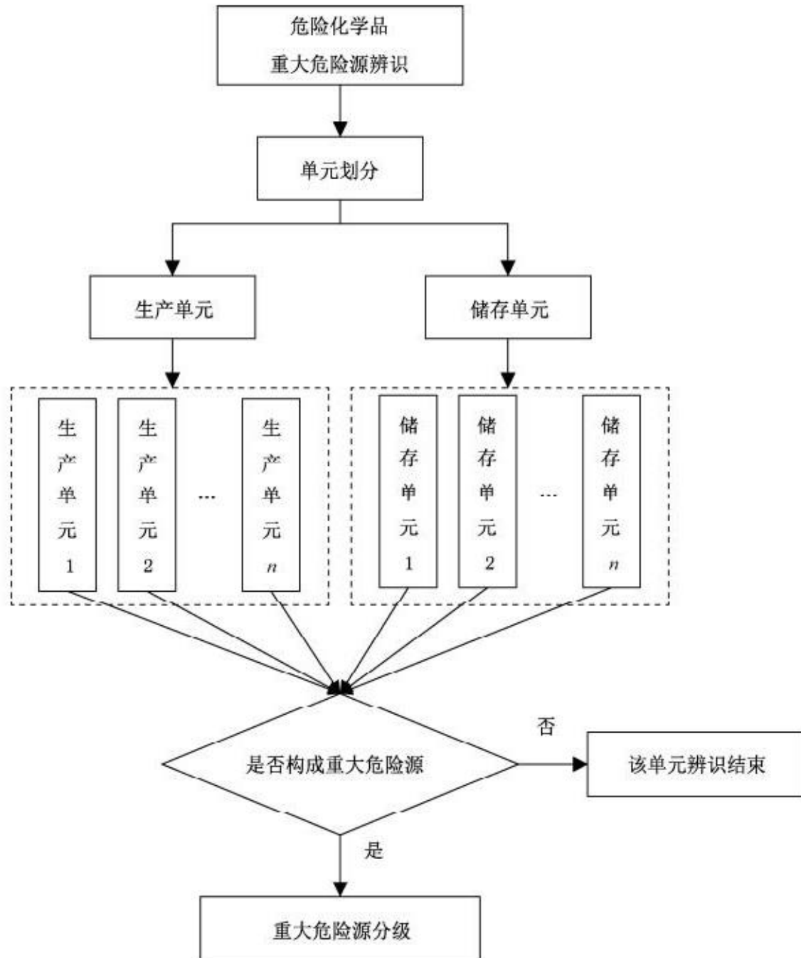
图 3.3-1 危险化学品重大危险源辨识流程图
