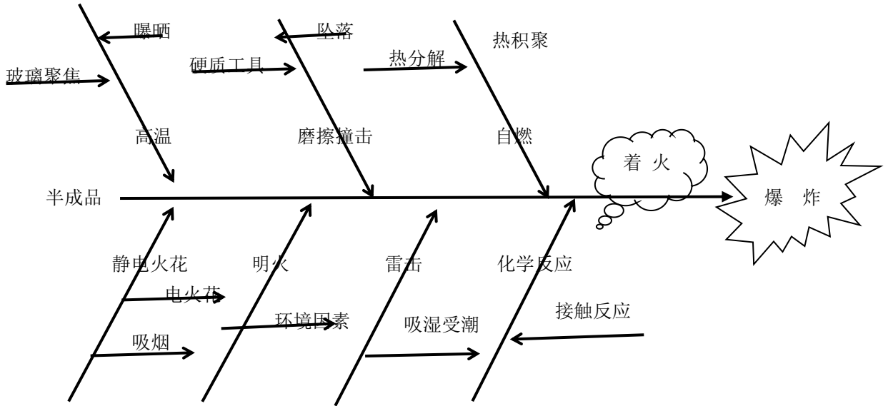
图 3-15-1 半成品燃烧、爆炸触发条件分析图
