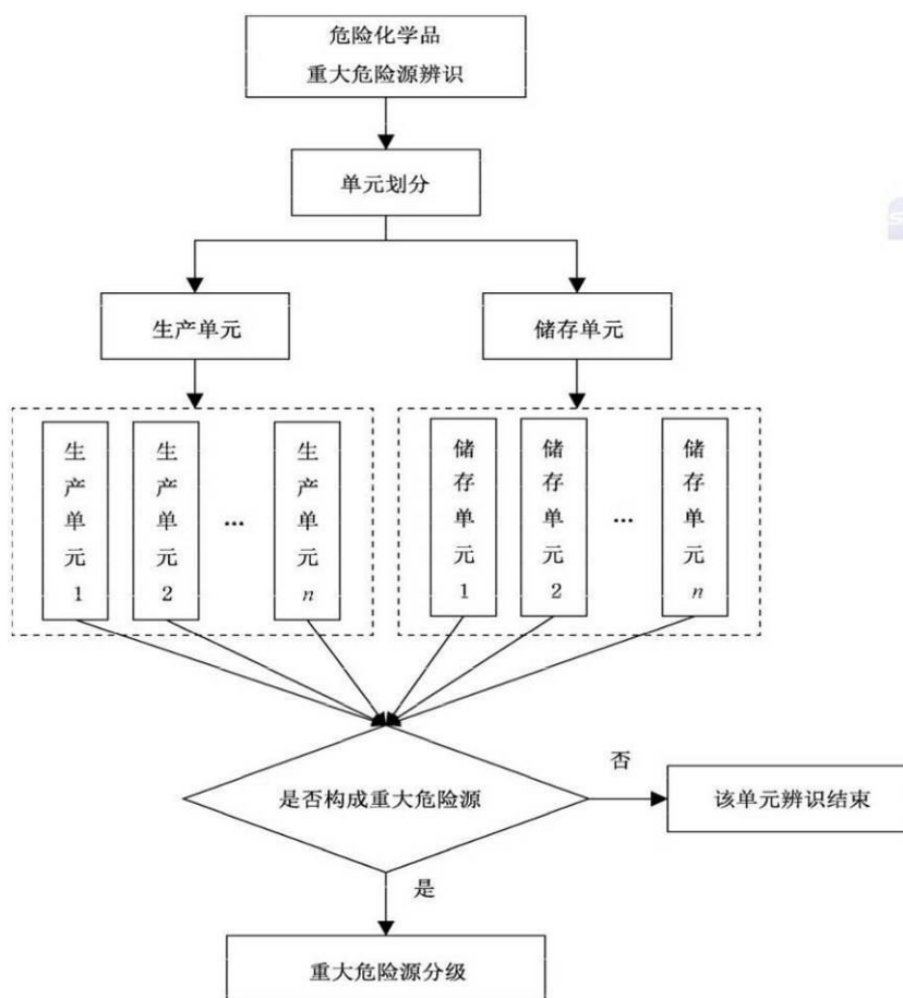
图 3.6-1 重大危险源辨识流程图
