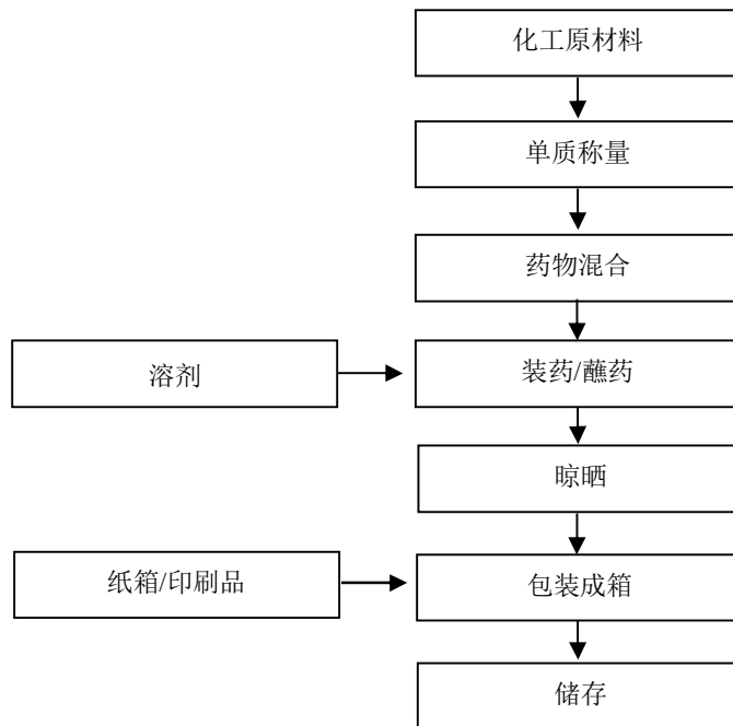
图 2-6：玩具类（线香型-晨光花）生产工艺流程图
