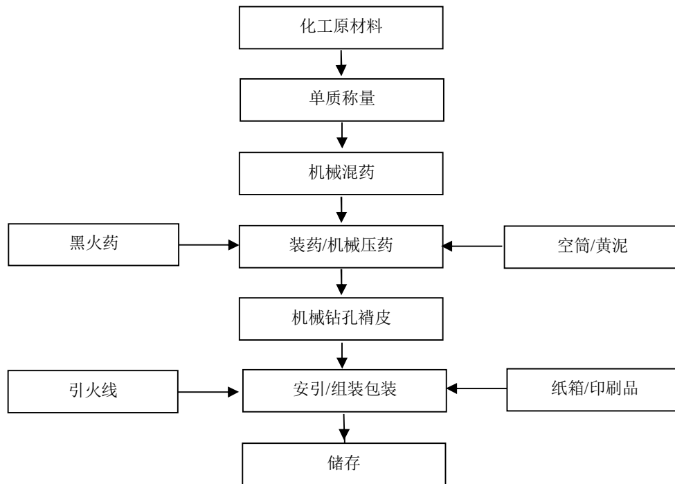
图 2-4：升空类（旋转升空烟花）/旋转类（如：大地花开）生产工艺流程图
