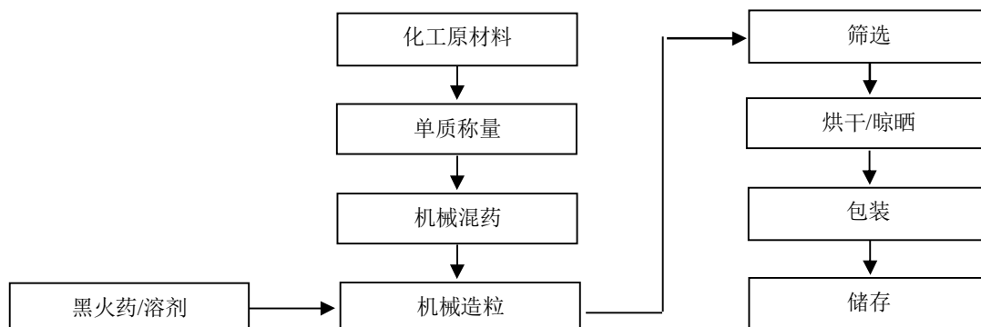
图 2-10：亮珠生产工艺流程图
