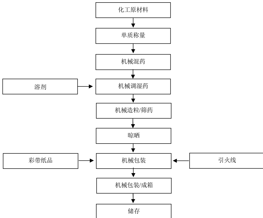
图 2-7：玩具类（玩具造型-糖果炮）生产工艺流程图
