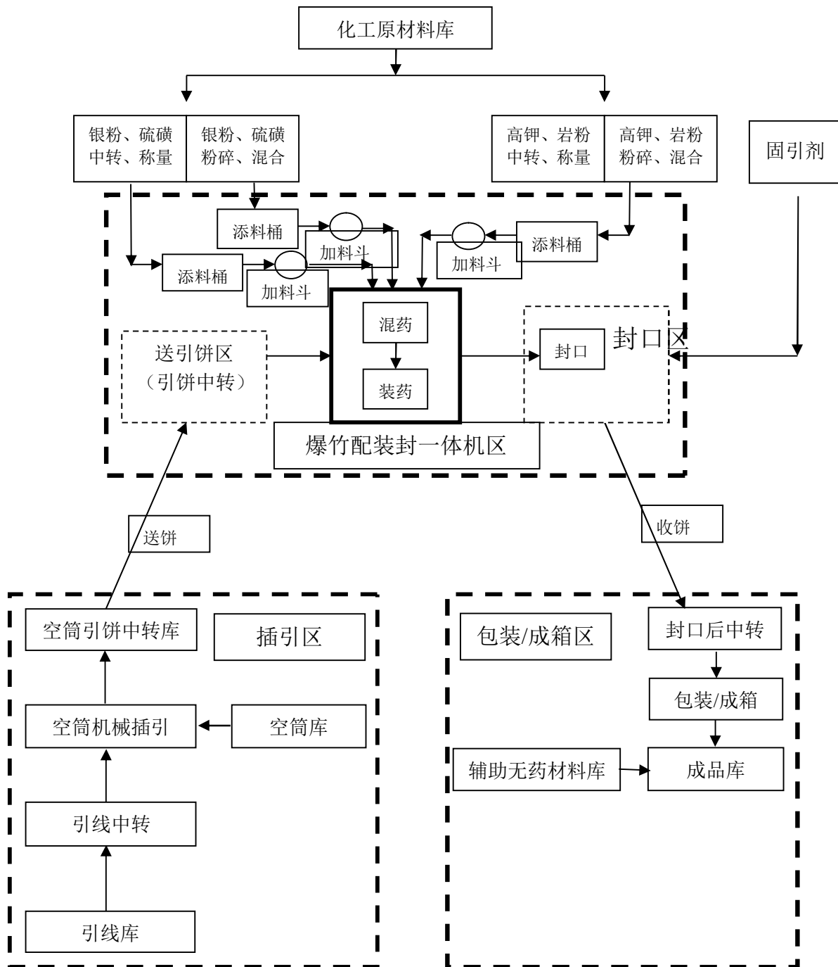
图 2-11：爆竹类（白药单响炮）生产工艺流程图
