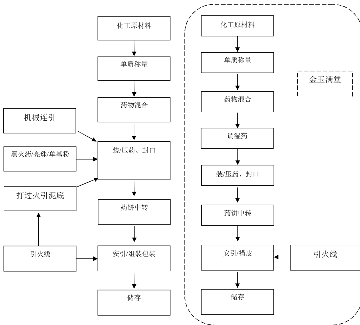
图 2-1：喷花类（花筒、金玉满堂）/玩具类（玩具造型）生产工艺流程图
