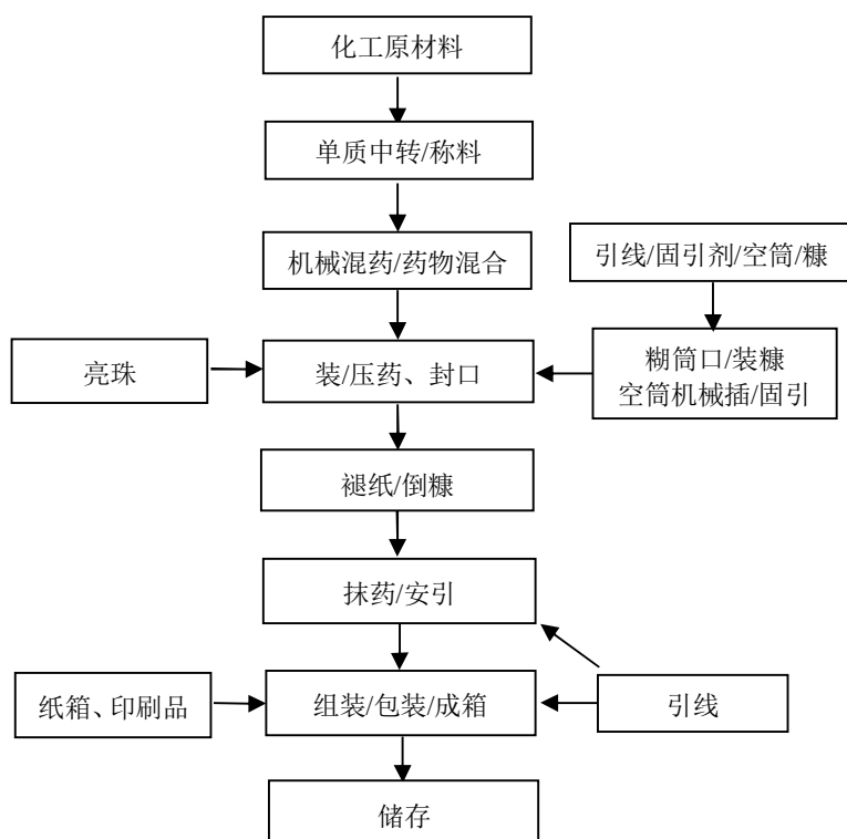
图 2-2：喷花类（闪光炮）生产工艺流程图
