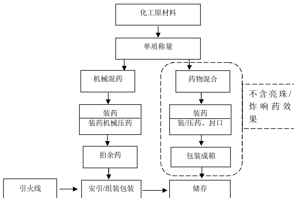
图 2-3：升空类（火箭）生产工艺流程图
