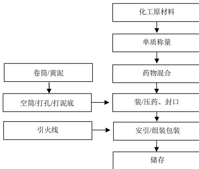
图 2-8：玩具类（烟雾型）生产工艺流程图
