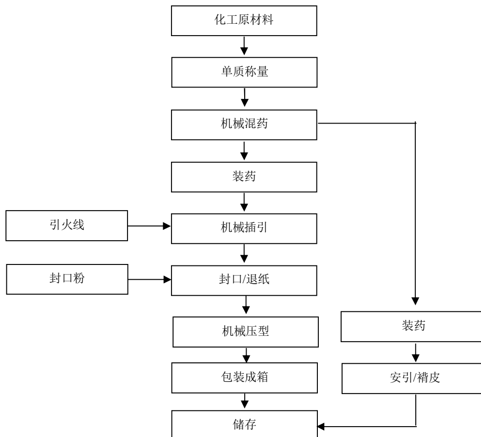
图 2-5：旋转类（彩菊）生产工艺流程图
