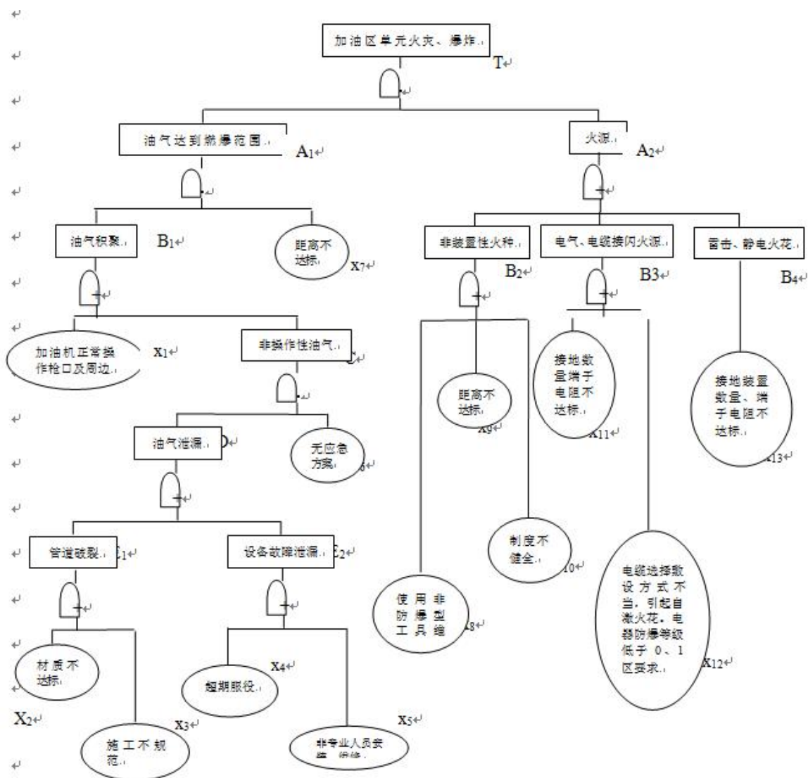
附图 3.2-1 油罐区火灾爆炸故障树
