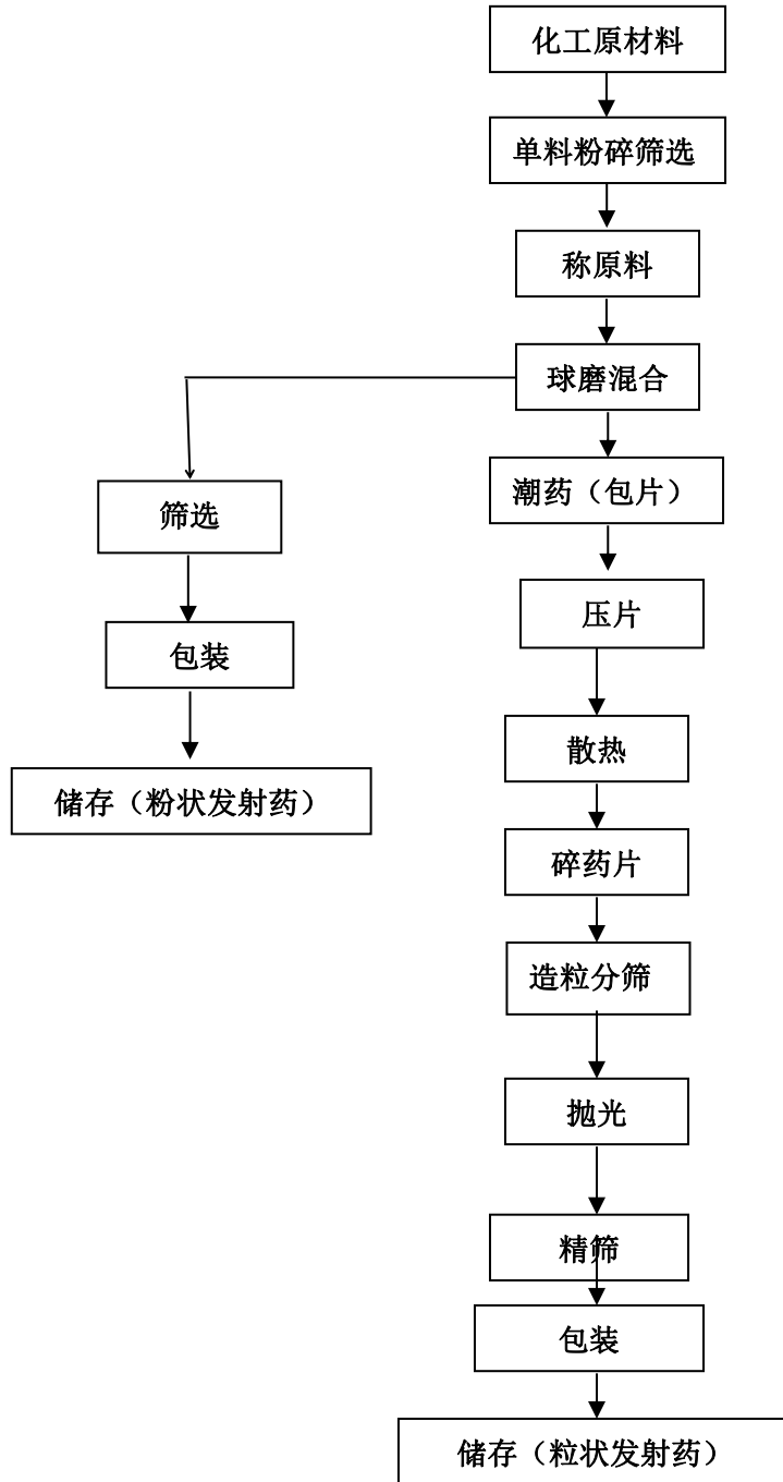
图 2-4-1 黑火药制造工艺流程图 (粉状、粒状发射药)
