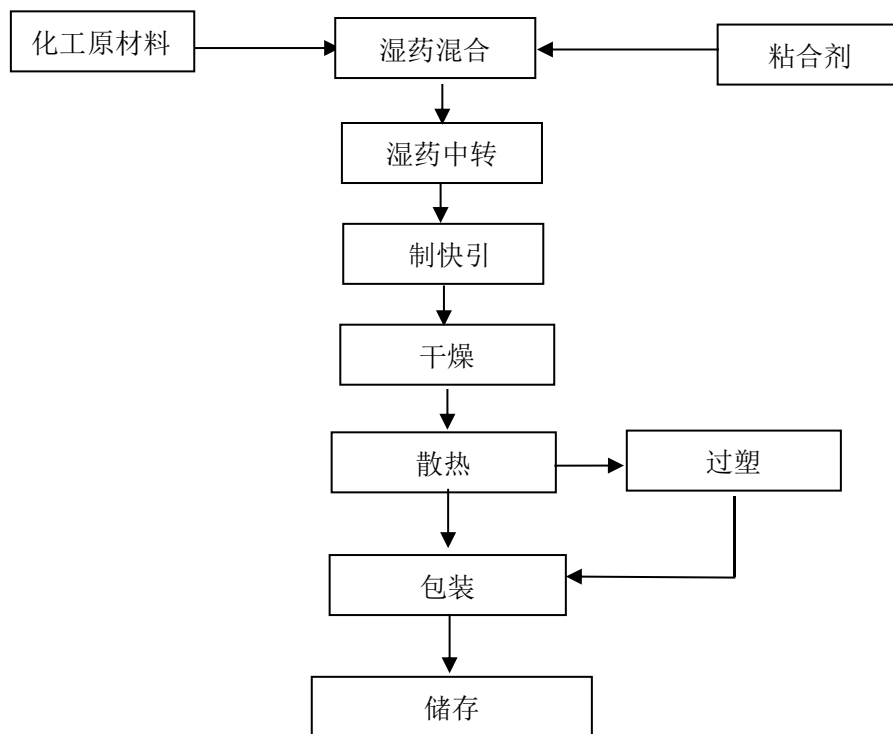
图 2-4-1 线引产品生产工艺流程图
