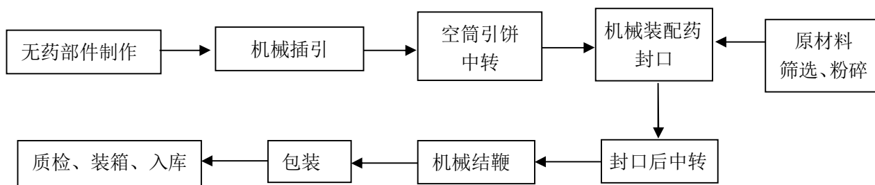
图 2-1：爆竹生产（插引）工艺流程图
