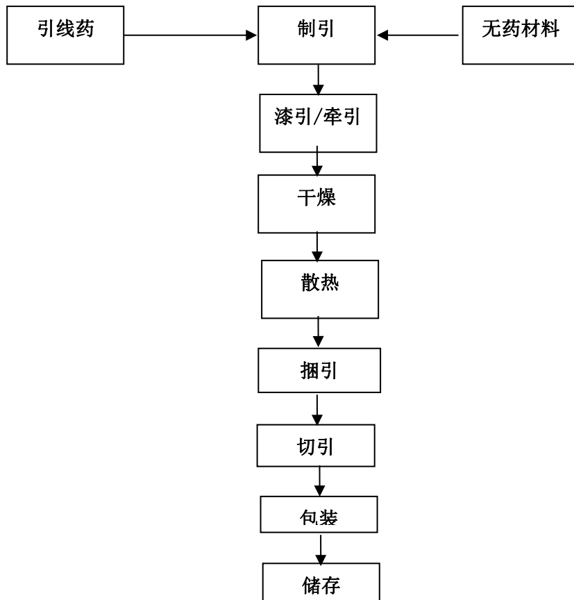
图 2-4-1 引药生产工艺流程图
