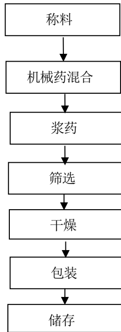
图 2-4-1 引药生产工艺流程图
