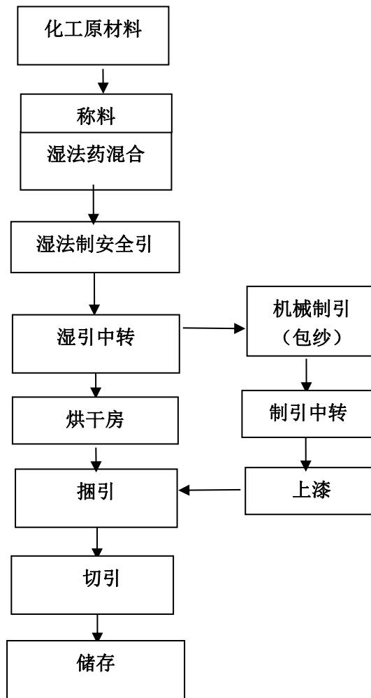
图 2-4-3 安全引（湿法）生产工艺流程
