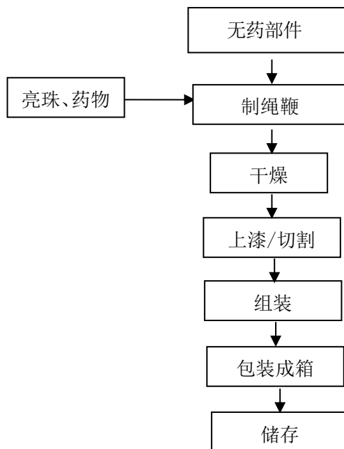
图 2-4-2 玩具类（线香型/绳鞭）生产工艺流程图
