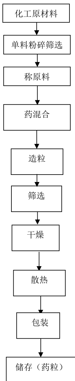
图 2-4-3 亮珠生产流程图
