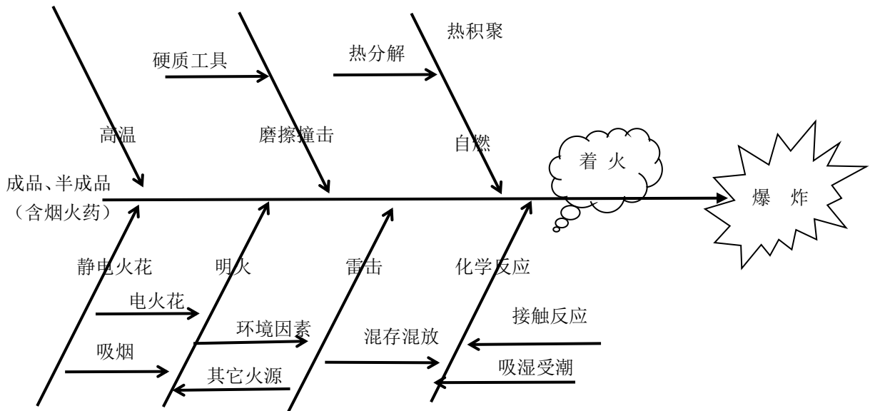
图 3-11-1 仓储场所爆炸的因果分析图
