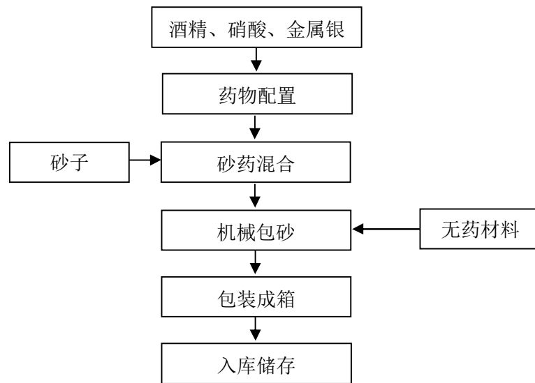
图 2.3-2：玩具类（摩擦型）生产工艺流程图
