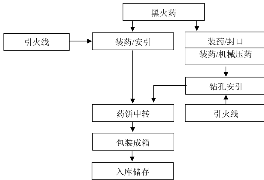
图 2.3-3：玩具类（玩具造型）生产工艺流程图
