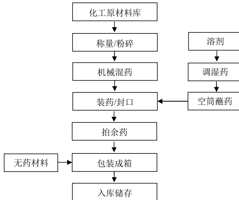
图 2.3-1：玩具类（线香型—晨光花）生产工艺流程图
