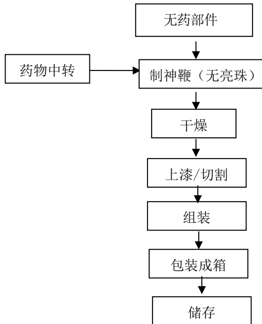
图 2-4-4 玩具类（线香型/神鞭）生产工艺流程图
