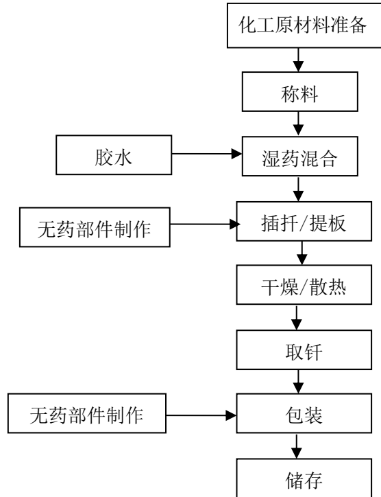
图 2-4-3 玩具类（线香型/电光型）生产工艺流程图
