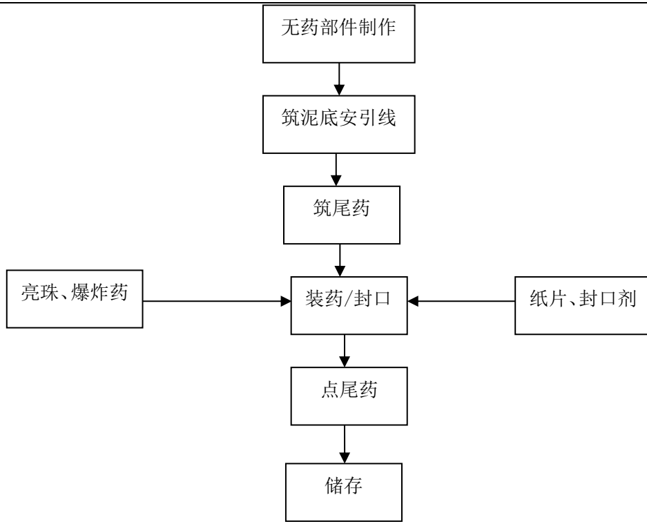
图 2-4-2 效果内筒生产流程
