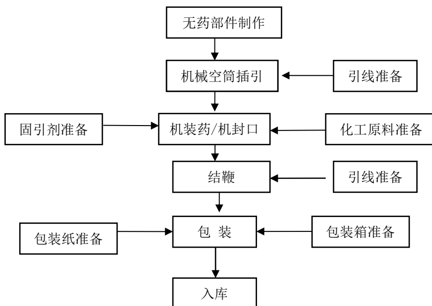
图 2-4 爆竹类产品生产工艺流程图
