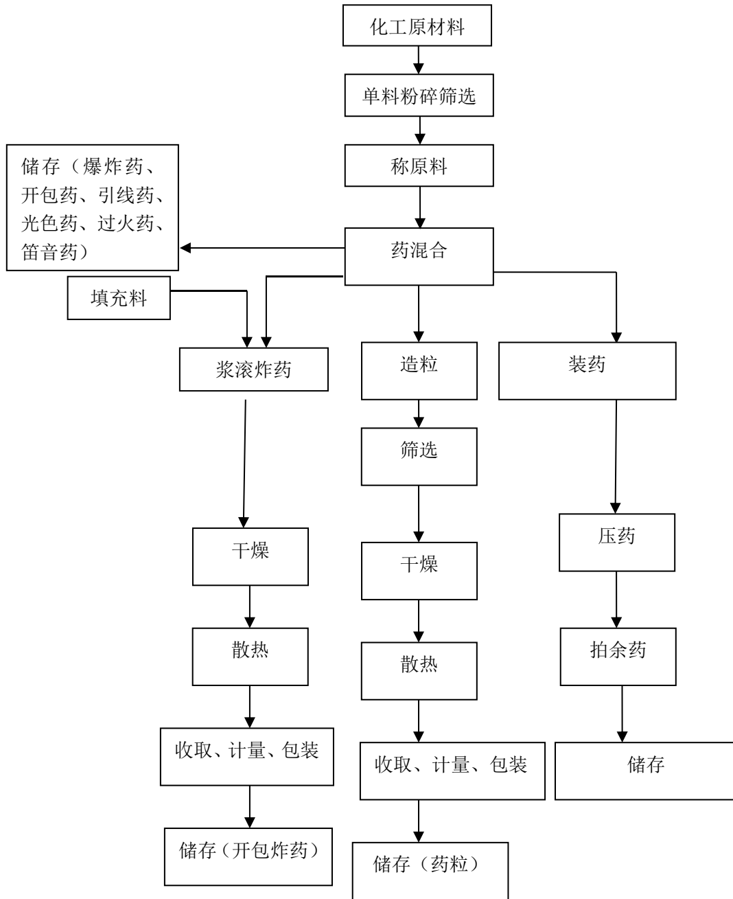
图 2-4-2 药物裸药效果件生产工艺流程图
