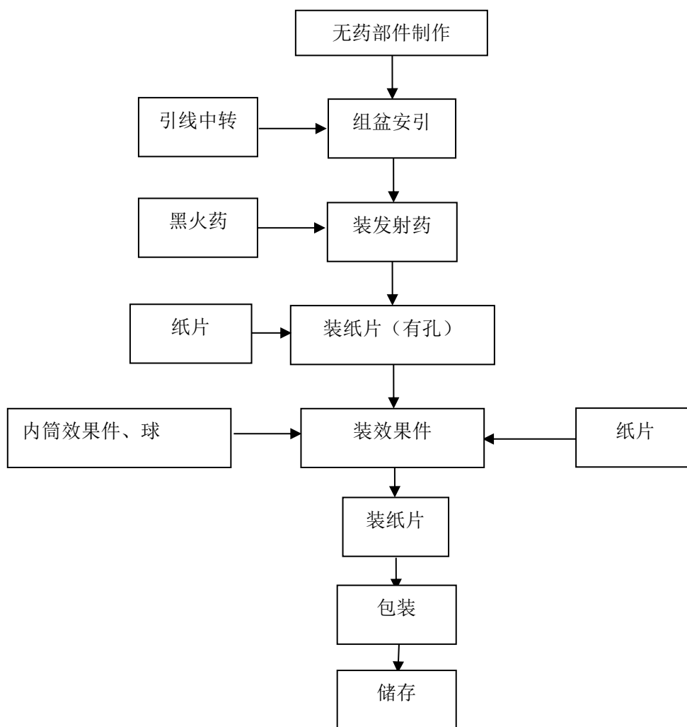
图 2-4-3 组合烟花产品生产工艺流程图
