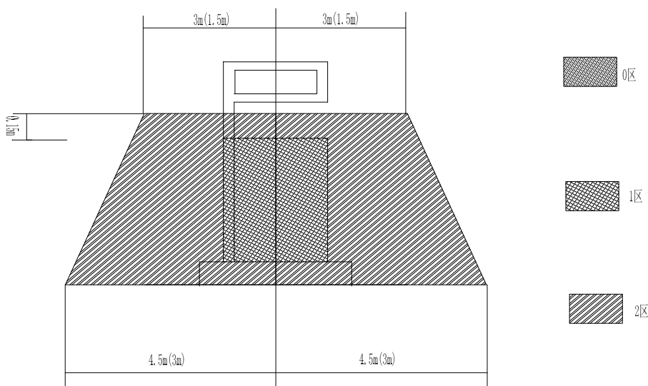
图 3.3-1 加油机爆炸危险区域划分
