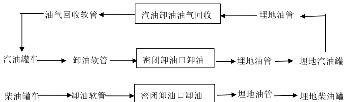
图2.6-1 汽车卸油工艺流程图
