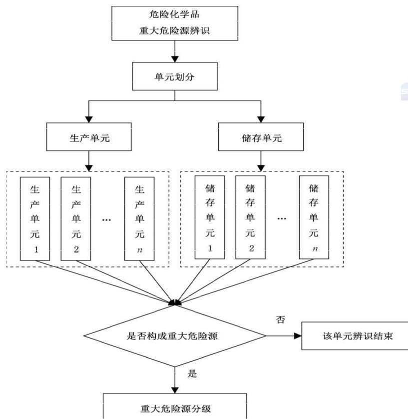
图 3.6-1 重大危险源辨识流程表
