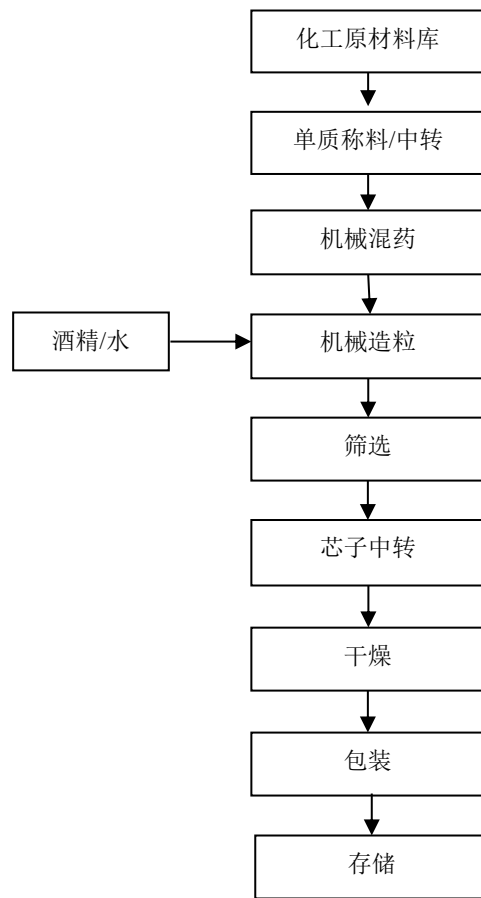
图 2-3：烟火药（亮珠）生产工艺流程图
