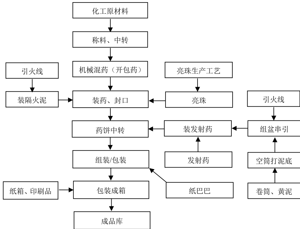
图 2-1 组合烟花类生产工艺流程图
