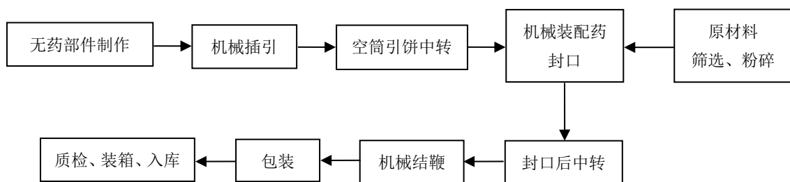
图 2-2 爆竹类生产工艺流程图
