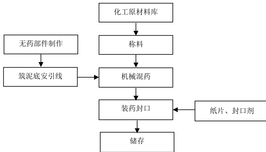
图 2-2：效果内筒工艺流程图
